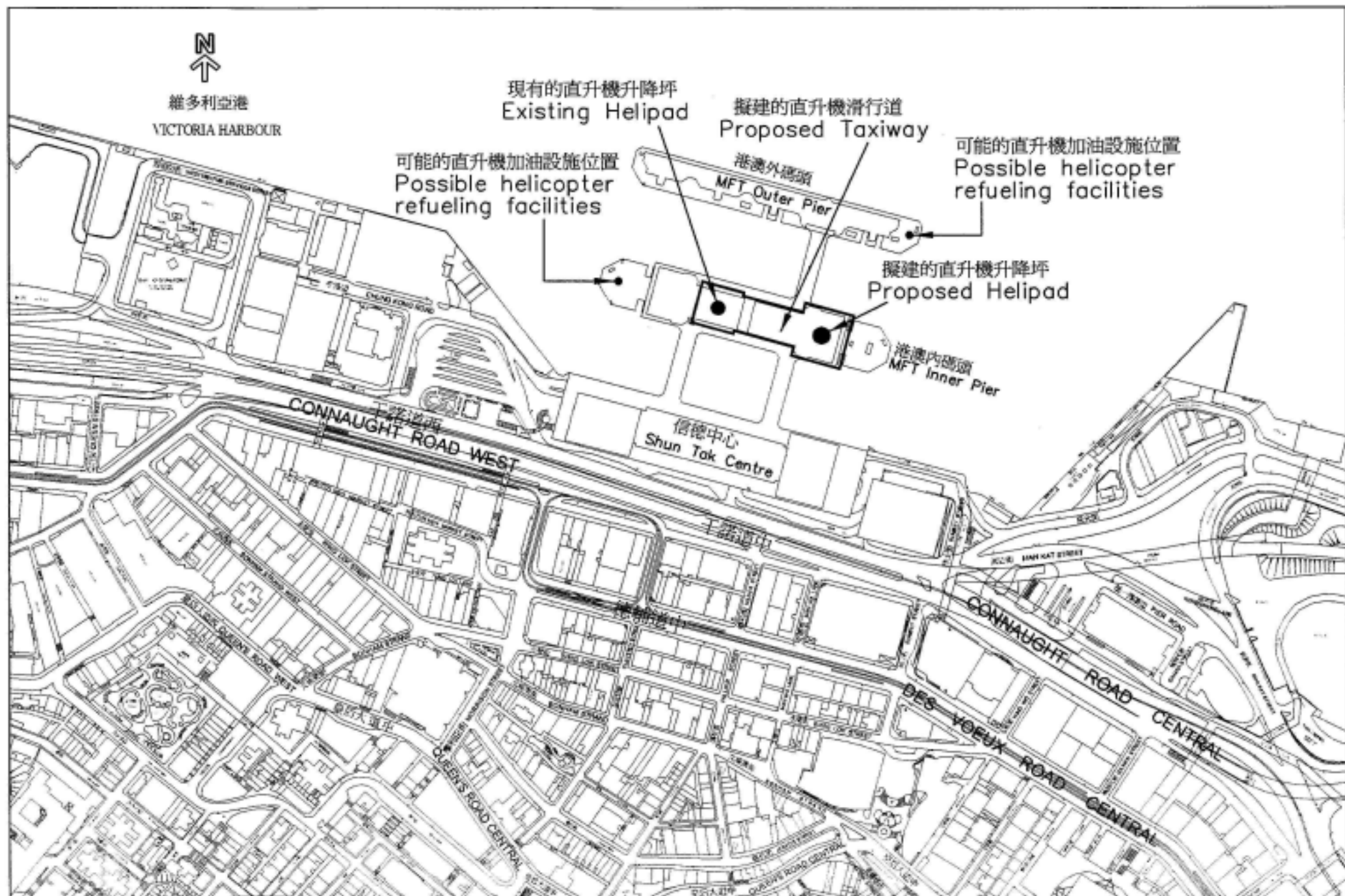
圖一 港澳碼頭現有和擬建的直升機場設施的位置
