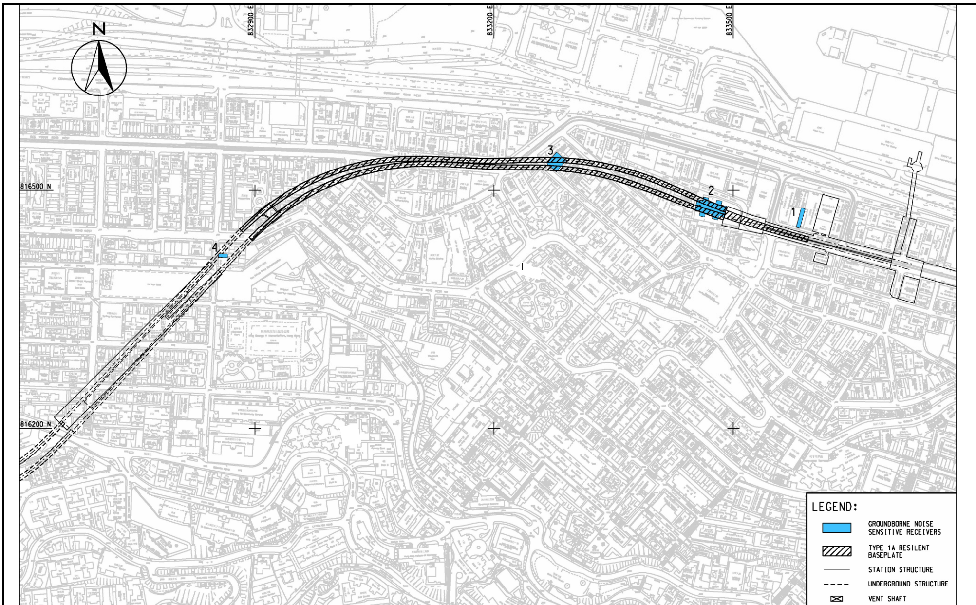
Figure 19: Rail Track Type 圖 19: 列車路軌類形
