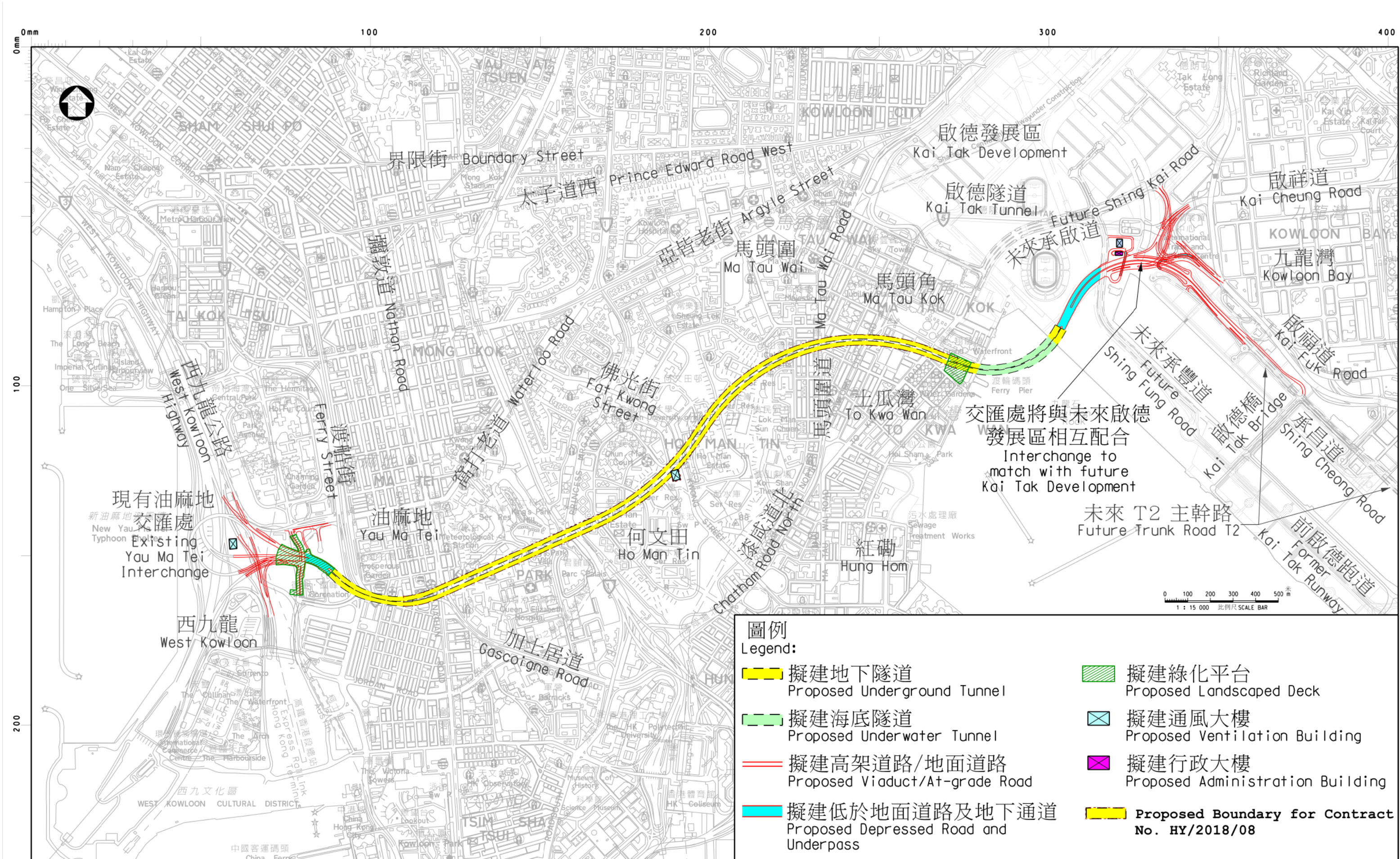
圖則名稱 plan title 工務計劃項目第6461TH號 中九龍幹線 - 主體工程 - 總平面圖 PWP Item No. 6461TH Central Kowloon Route - Main Works - General Layout Plan
