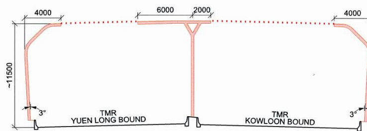
SECTION 14-14 SEMI-ENCLOSURE NM 21 (N.T.S.)
