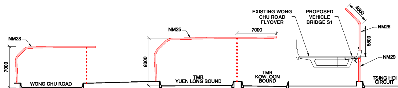
SECTION 19-19 BARRIER NM29 (N.T.S.)
