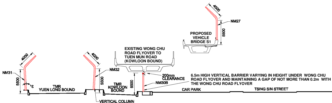
SECTION 20-20 BARRIER NM30B (N.T.S.)
