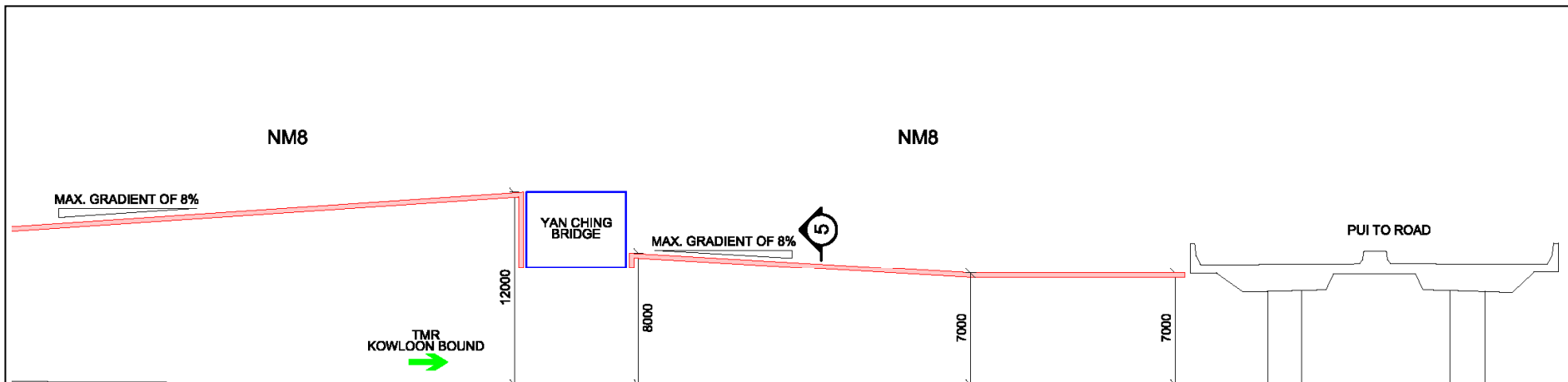
LONGITUDINAL SECTION ALONG TMR KOWLOON BOUND AT NM8 (N.T.S.)
