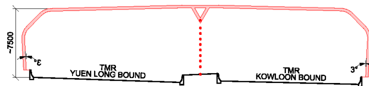
SECTION 5-5 FULL ENCLOSURE NM 8 (N.T.S.)
