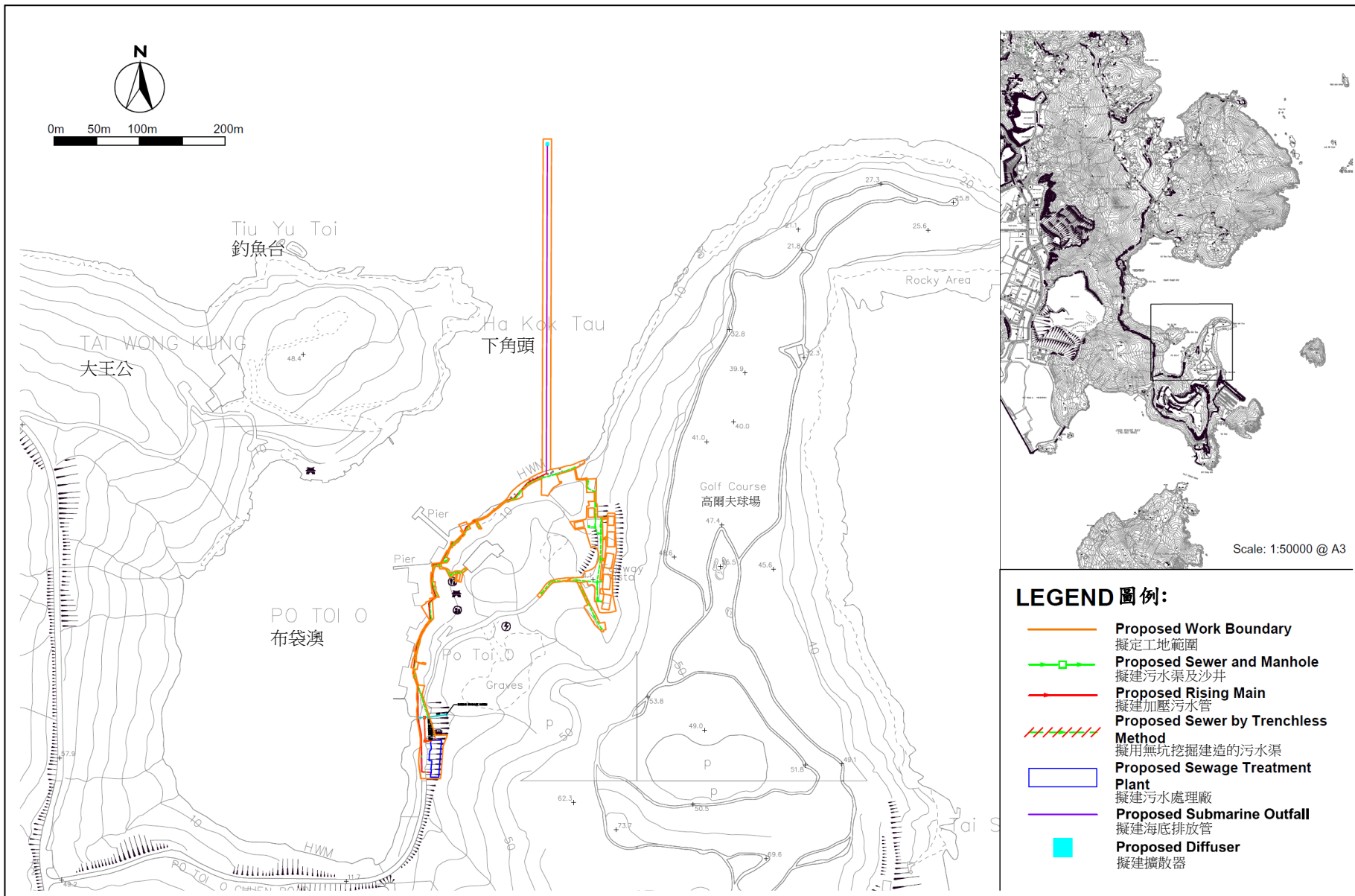
Project Title: Port Shelter Sewerage, Stage 3 – Sewerage Works at Po Toi O 工程項目名稱：牛尾海污水收集系統第三階段 - 布袋澳污水收集系統工程 Layout Plan of Proposed Sewerage Works 污水收集系統工程平面圖
