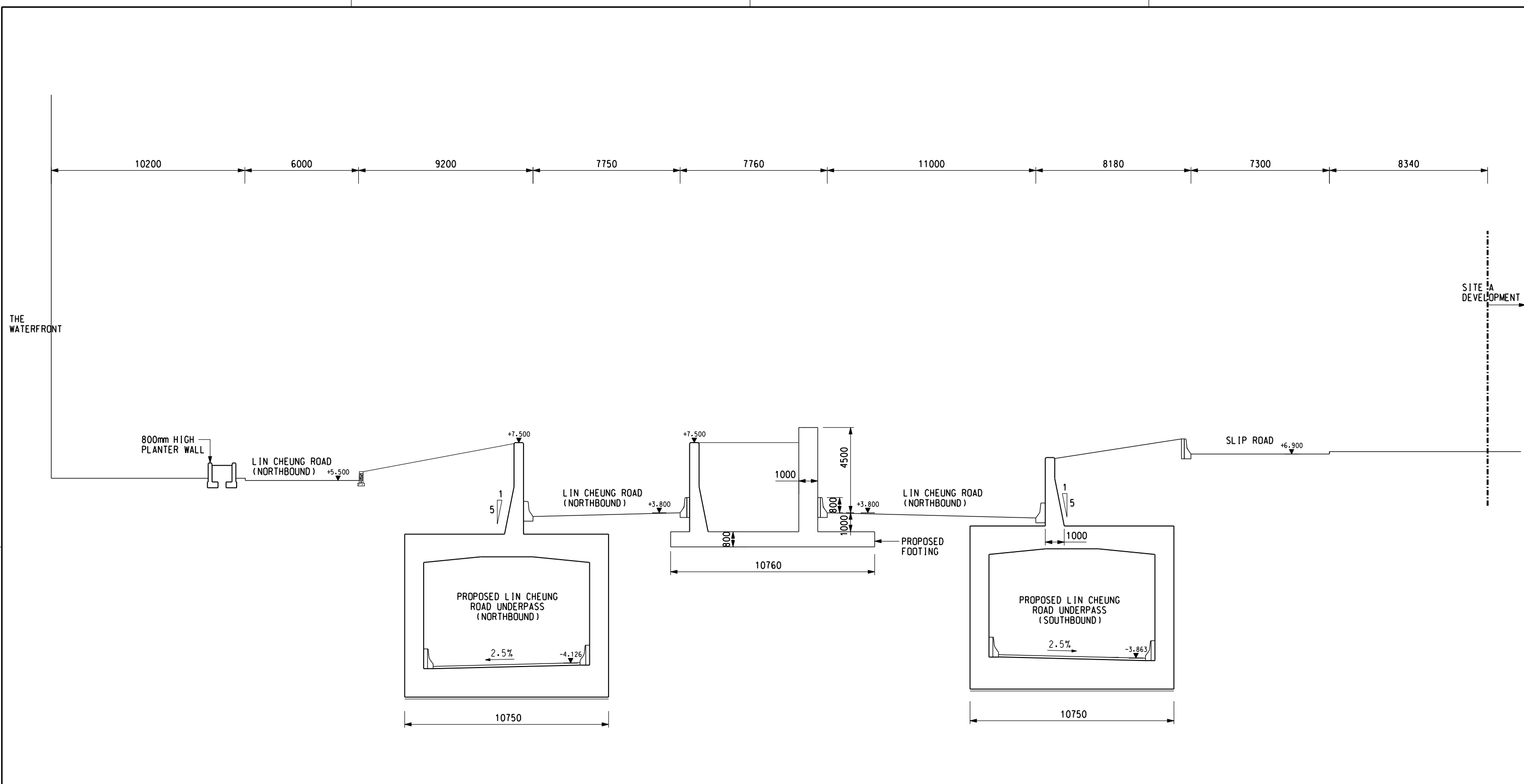
SECTION 6 SCALE 1 : 200
