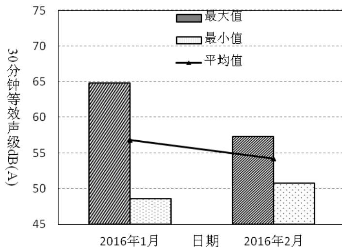
图4-20 香港较寮村2016年1月~2月昼间噪音变化趋势
