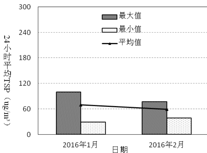
图3-10 2016年1月至2月香港较寮村24小时TSP变化趋势
