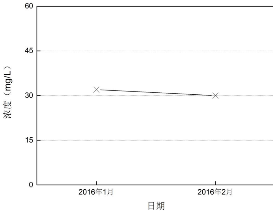
图5-10 深圳河砂石传送带监测点16年1月~2月COD变化趋势图
