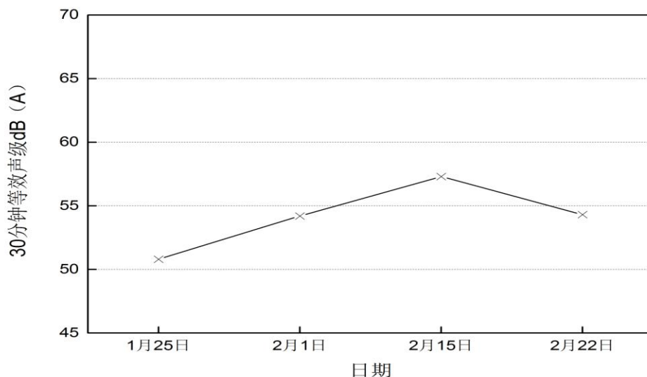
图4-10 2016年2月香港较寮村昼夜噪音声级变化趋势
