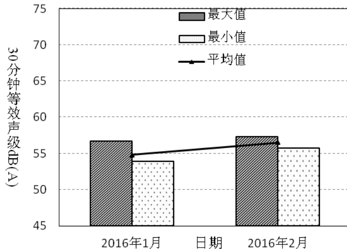
图4-19 香港打鼓岭村2016年1月~2月昼间噪音变化趋势
