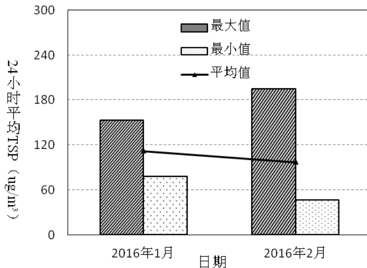
图3-9 2016年1月至2月罗芳村和幼儿园24小时TSP变化趋势
