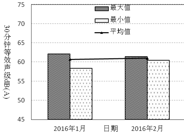
图4-17 鹏兴花园2016年1月~2月昼间噪音变化趋势
