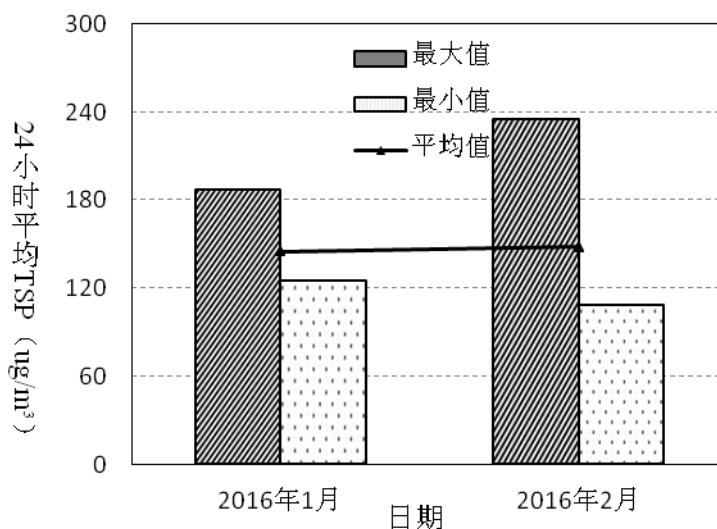
图3-8 2016年1月至2月曦龙山庄24小时TSP变化趋势
