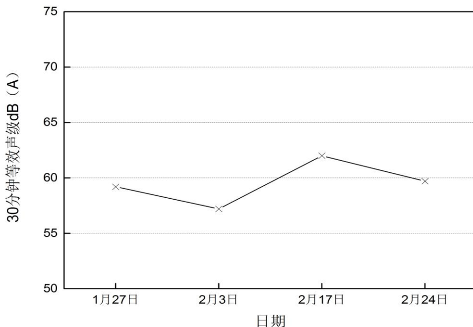
图4-2 2016年2月罗芳村小学和幼儿园昼夜噪音声级变化趋势
