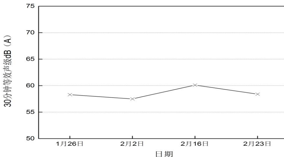
图4-4 2016年2月罗湖区委党校昼夜噪音声级变化趋势
