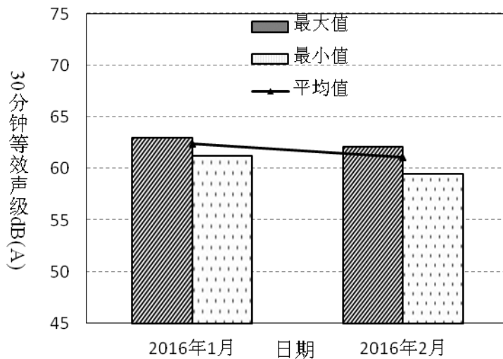
图4-13 罗芳村2016年1月~2月昼间噪音变化趋势
