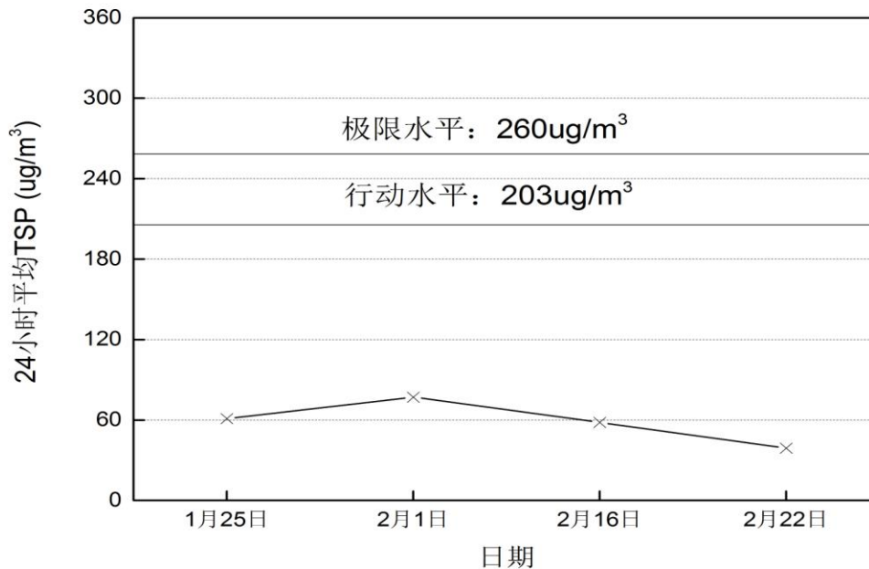
图3-5 2016年2月较寮村24小时平均TSP变化趋势
