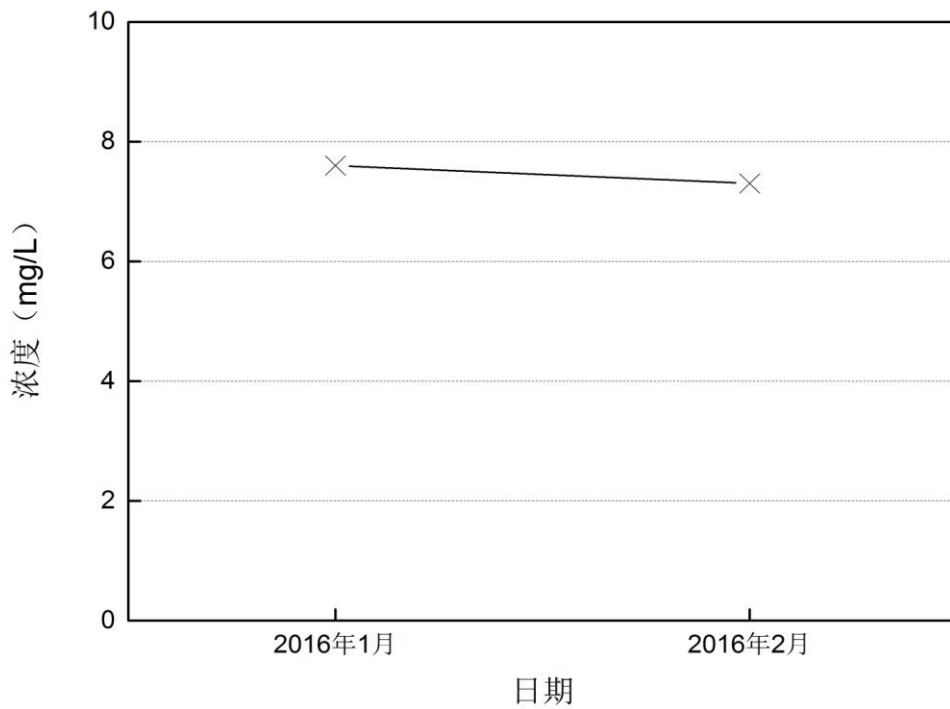
图5-9 深圳河砂石传送带监测点16年1月~2月DO变化趋势图
