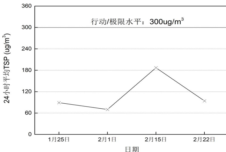
图3-2 2016年2月鹏兴花园24小时平均TSP变化趋势
