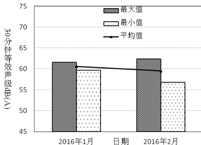
图4-18 港莲一村2016年1月~2月昼间噪音变化趋势
