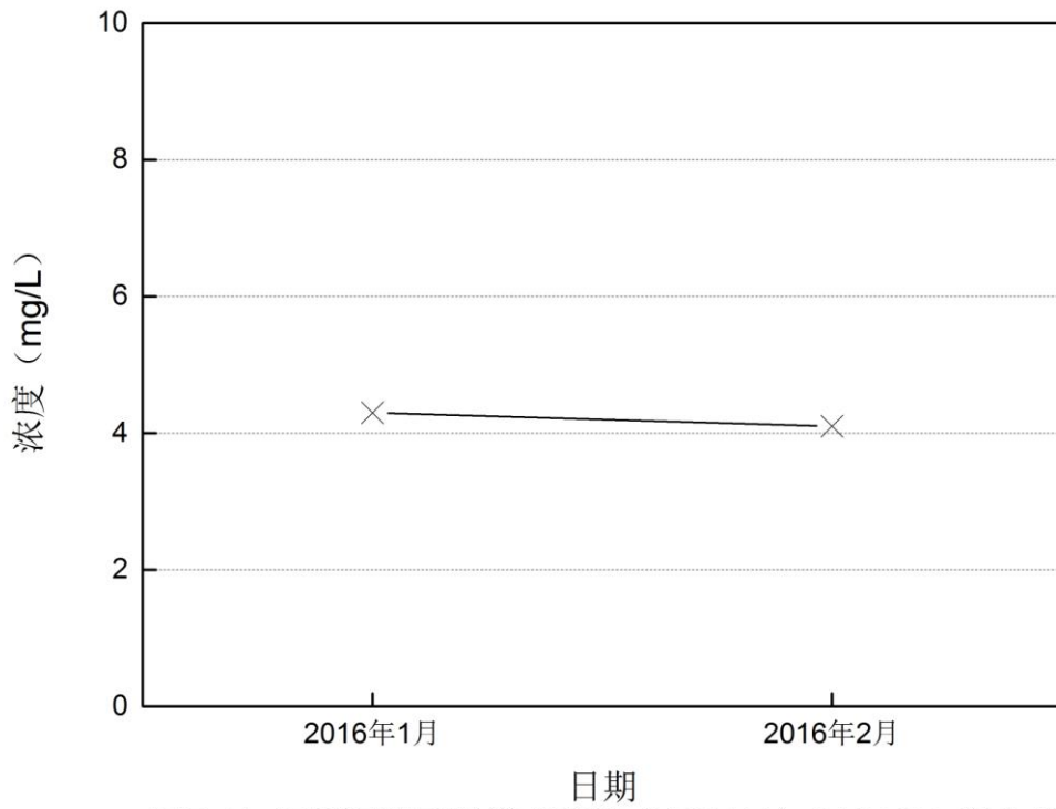
图5-11 深圳河砂石传送带监测点16年1月~2月BOD 5 变化趋势图
