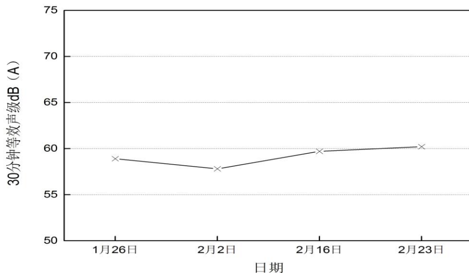
图4-5 2016年2月曦龙山庄昼夜噪音声级变化趋势
