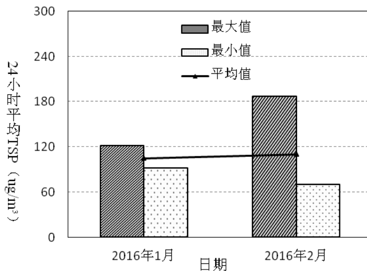
图3-7 2016年1月至2月鹏兴花园24小时TSP变化趋势
