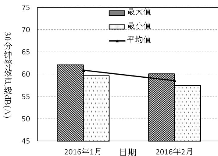
图4-14 罗湖区委党校2016年1月~2月昼间噪音变化趋势
