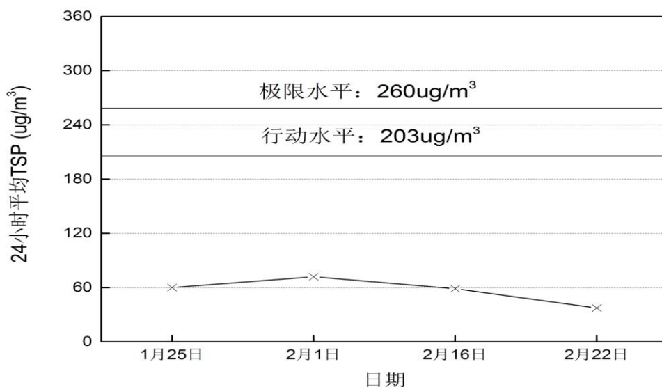
图3-6 2016年2月较寮村24小时平均TSP变化趋势
