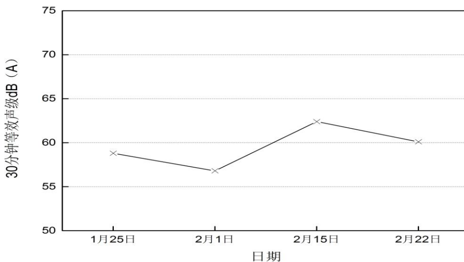
图4-8 2016年2月港莲一村昼夜噪音声级变化趋势
