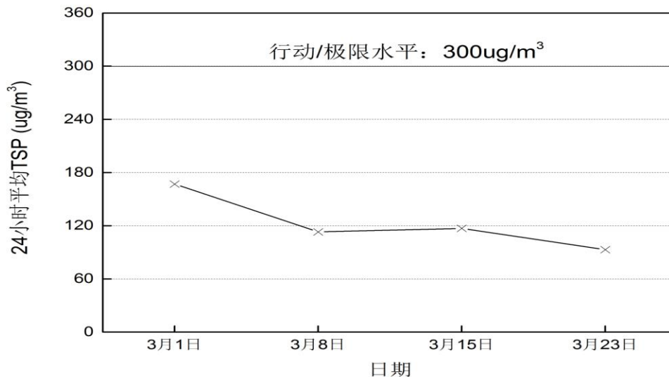
图3-3 2016年3月曦龙山庄24小时平均TSP变化趋势
