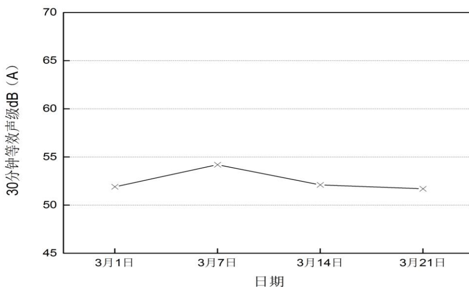
图4-10 2016年3月香港较寮村昼夜噪音声级变化趋势
