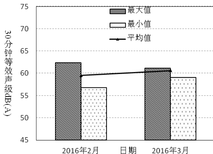
图4-18 港莲一村2016年2月~3月昼间噪音变化趋势
