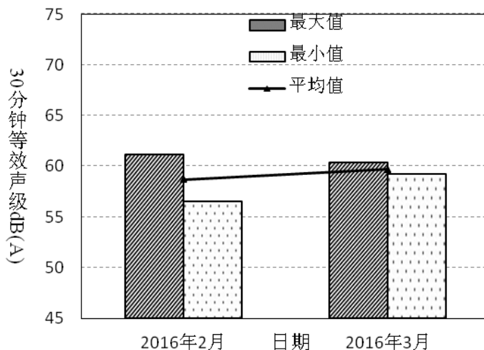
图4-11 峰度天下2016年2月~3月昼间噪音变化趋势
