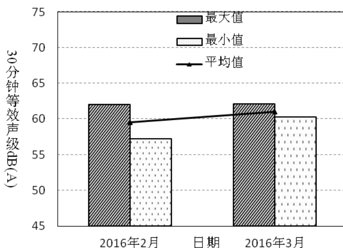
图4-12 罗芳村小学和幼儿园2016年2月~3月昼间噪音变化趋势
