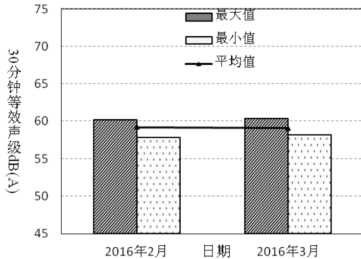
图4-15 曦龙山庄2016年2月~3月昼间噪音变化趋势
