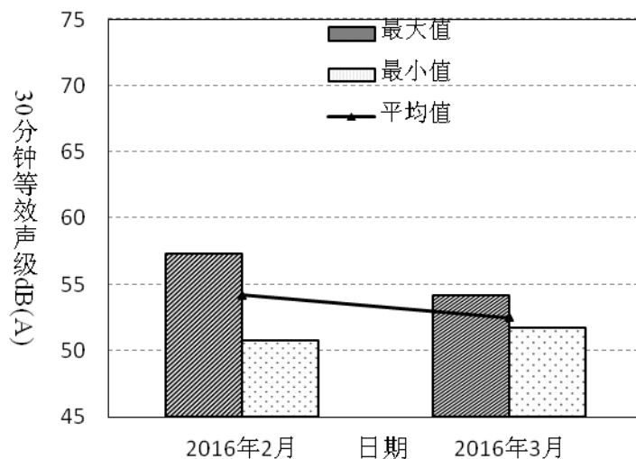
图4-20 香港较寮村2016年2月~3月昼间噪音变化趋势
