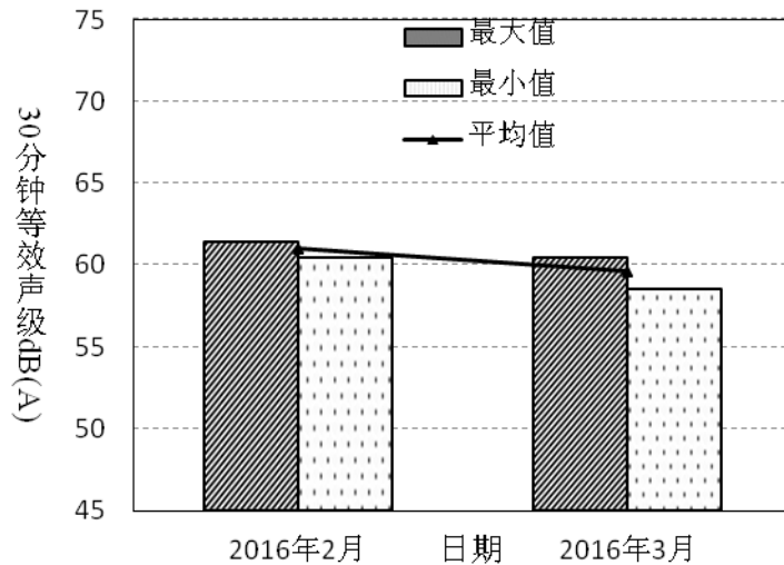
图4-17 鹏兴花园2016年2月~3月昼间噪音变化趋势
