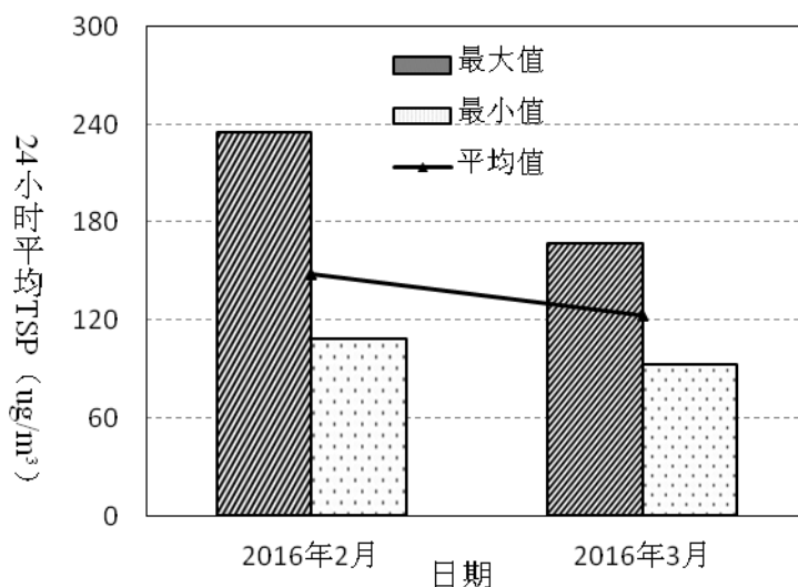
图3-8 2016年2月至3月曦龙山庄24小时TSP变化趋势
