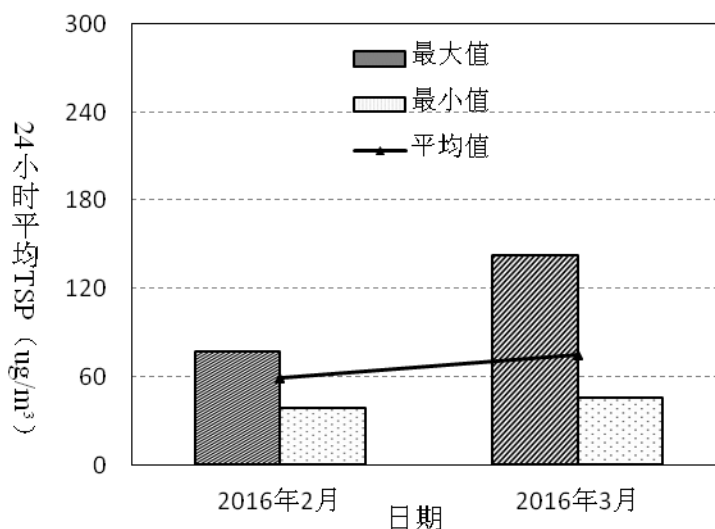
图3-10 2016年2月至3月香港较寮村24小时TSP变化趋势
