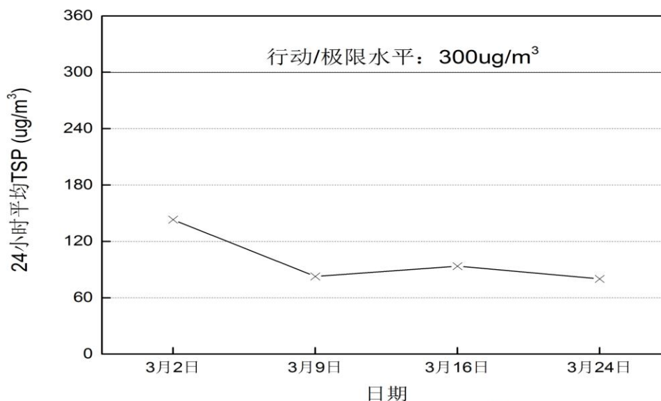
图3-4 2016年3月罗芳村和幼儿园24小时平均TSP变化趋势
