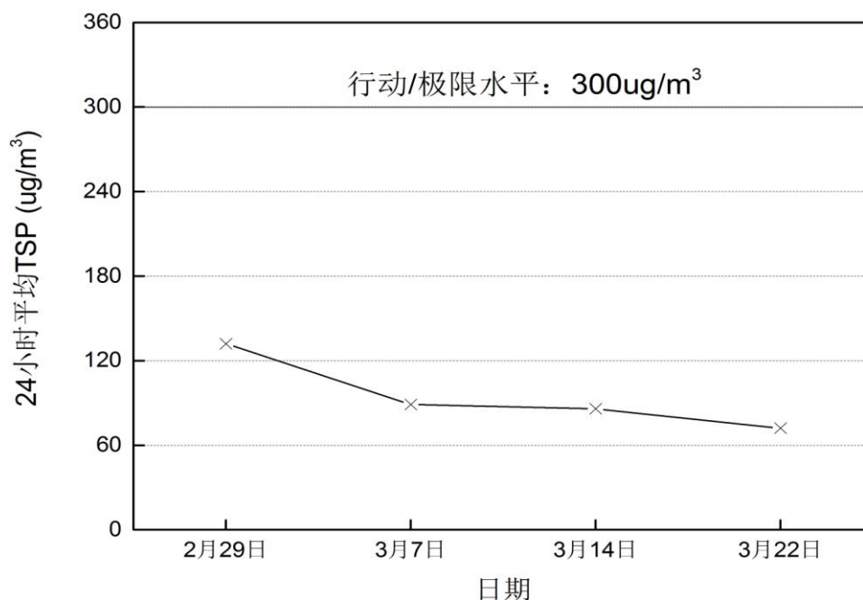
图3-2 2016年3月鹏兴花园24小时平均TSP变化趋势
