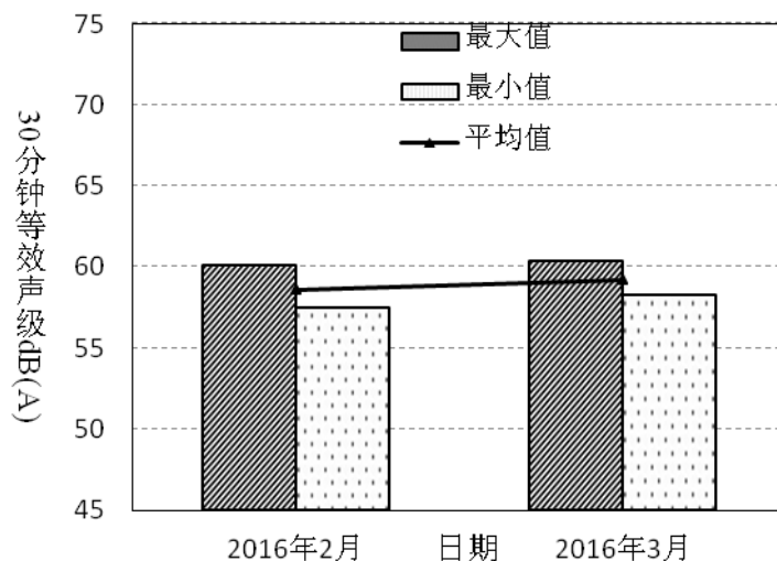
图4-14 罗湖区委党校2016年2月~3月昼间噪音变化趋势
