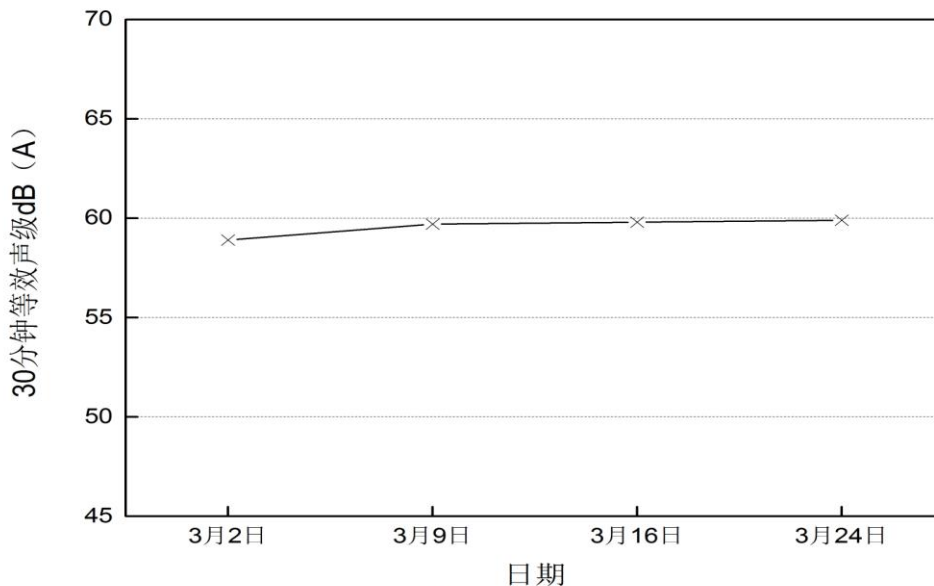
图4-3 2016年3月罗芳村昼夜噪音声级变化趋势
