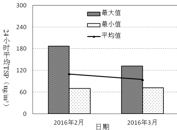
图3-7 2016年2月至3月鹏兴花园24小时TSP变化趋势
