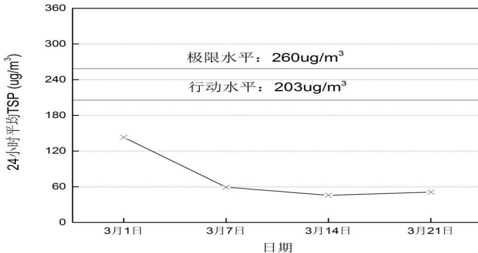
图3-5 2016年3月较寮村24小时平均TSP变化趋势
