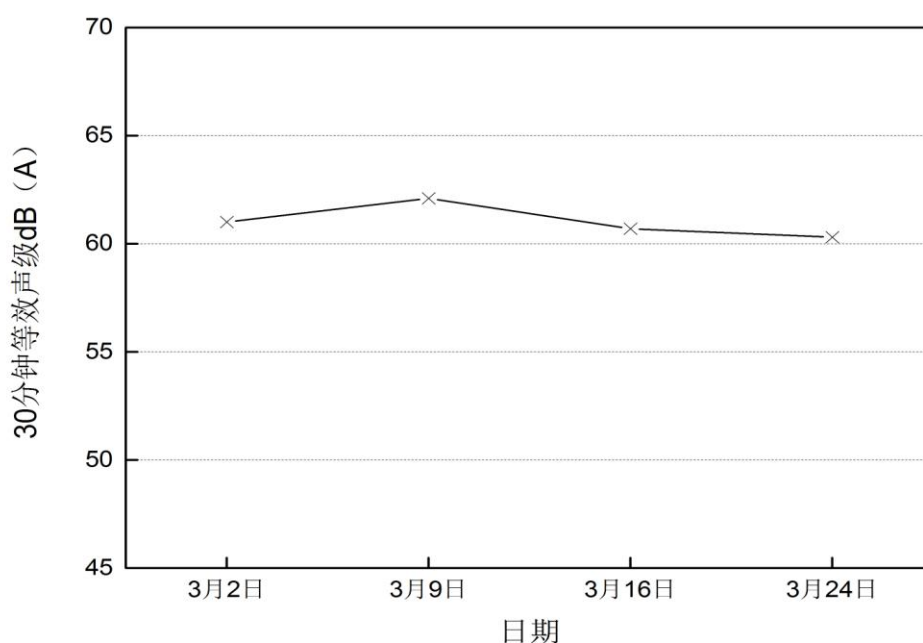
图4-2 2016年3月罗芳村小学和幼儿园昼夜噪音声级变化趋势
