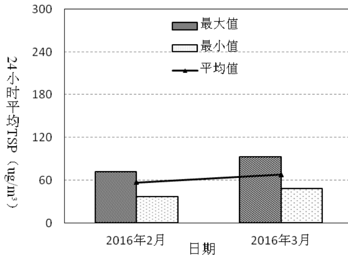
图3-11 2016年2月至3月香港松园下村24小时TSP变化趋势
