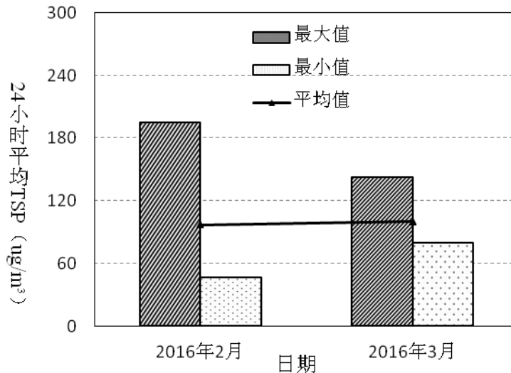
图3-9 2016年2月至3月罗芳村和幼儿园24小时TSP变化趋势
