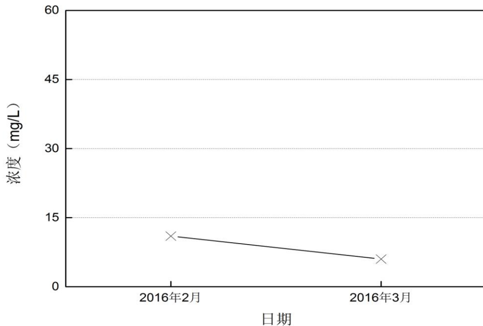
图5-2 深圳河砂石传送带监测点16年2月~3月SS变化趋势图
