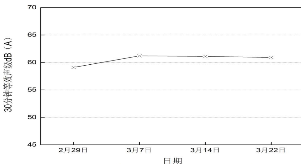
图4-8 2016年3月港莲一村昼夜噪音声级变化趋势
