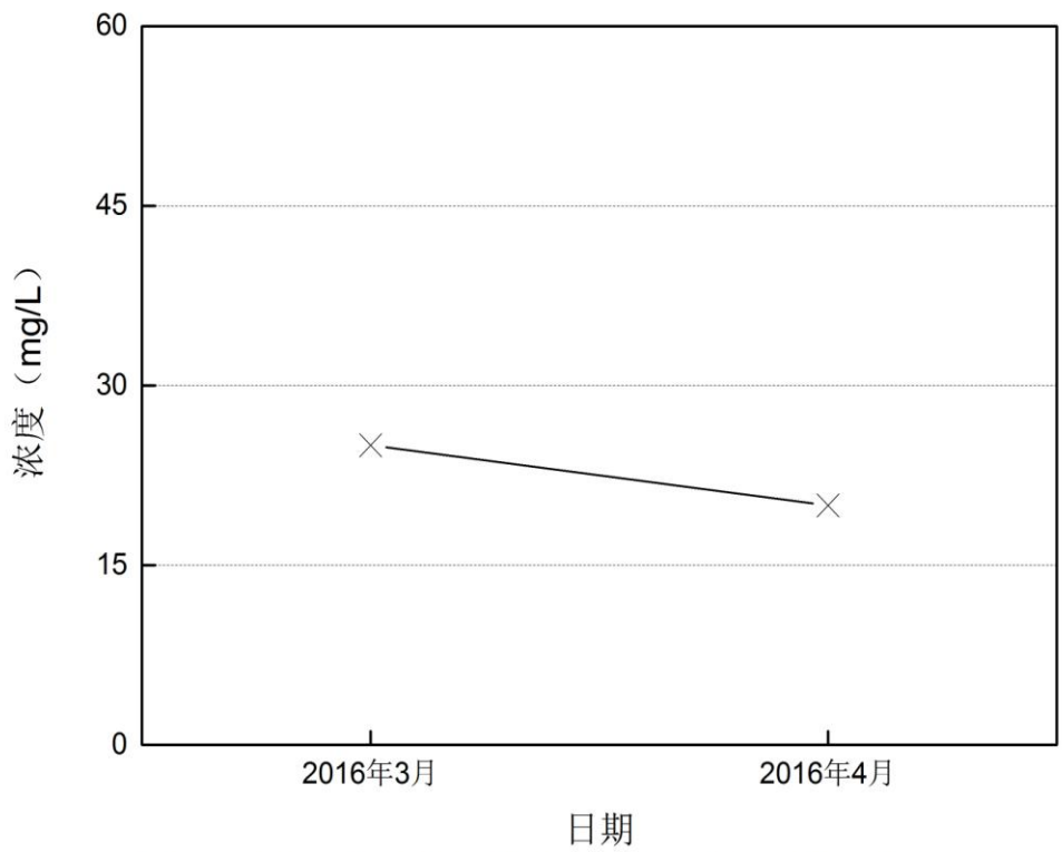
图5-4 深圳河长岭村监测点16年3月~4月COD变化趋势图
