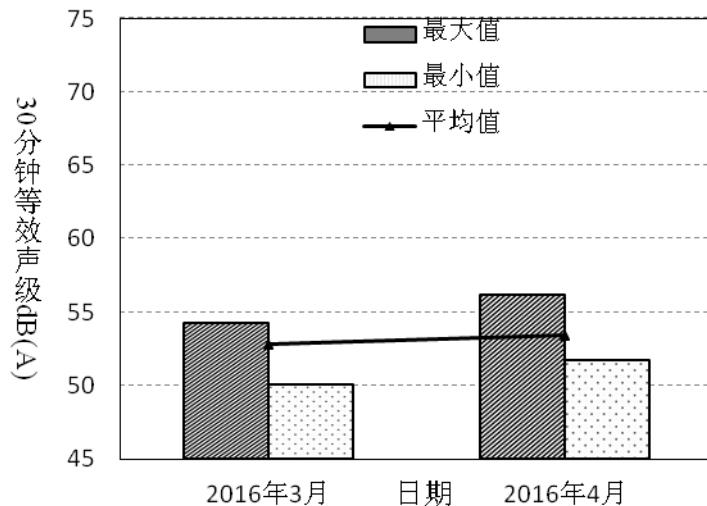
图4-19 香港打鼓岭村2016年3月~4月昼间噪音变化趋势
