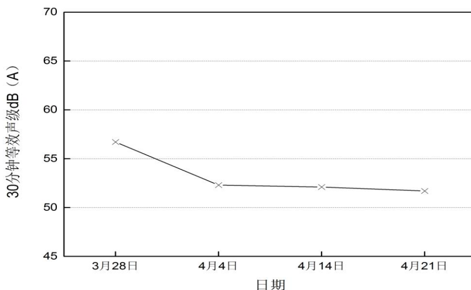
图4-10 2016年4月香港较寮村昼夜噪音声级变化趋势
