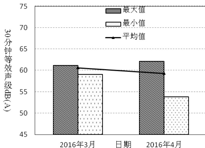
图4-18 港莲一村2016年3月~4月昼间噪音变化趋势
