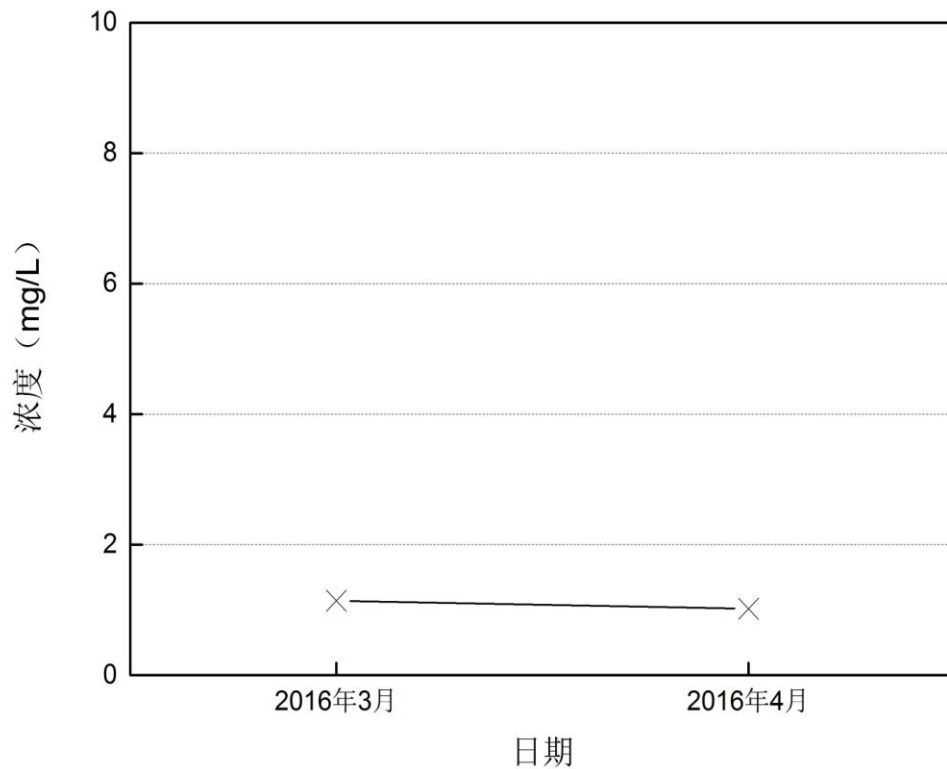
图5-6 深圳河长岭村监测点16年3月~4月氨氮变化趋势图
