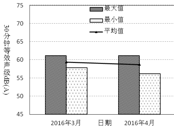
图4-16 观澜国际2016年3月~4月昼间噪音变化趋势
