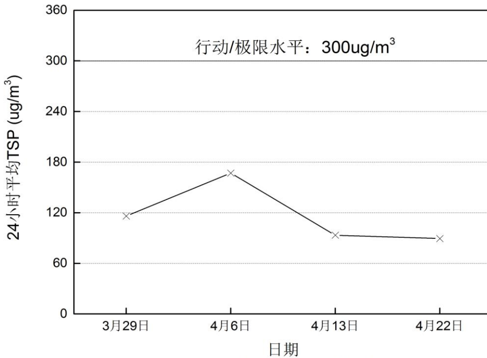
图3-3 2016年4月曦龙山庄24小时平均TSP变化趋势
