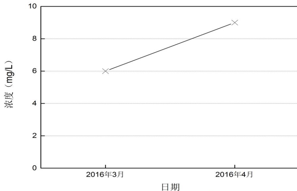
图5-2 深圳河砂石传送带监测点16年3月~4月SS变化趋势图
