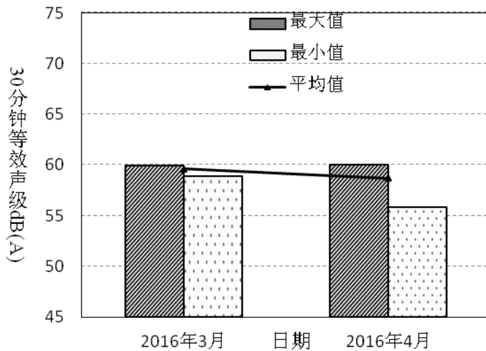
图4-13 罗芳村2016年3月~4月昼间噪音变化趋势
