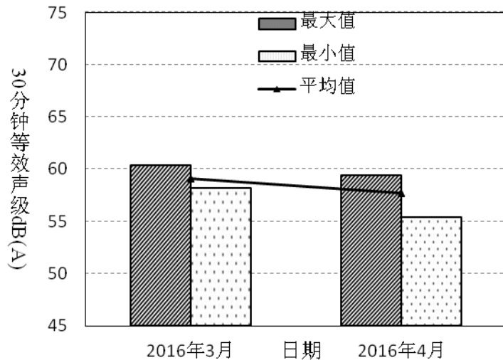
图4-15 曦龙山庄2016年3月~4月昼间噪音变化趋势
