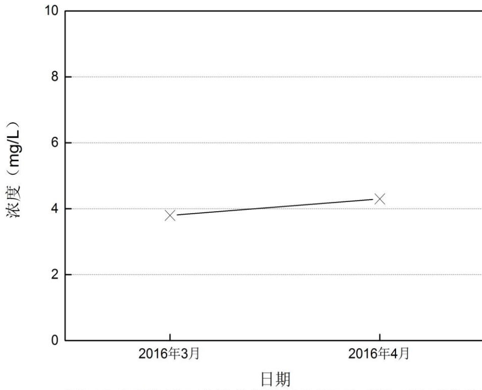
图5-11 深圳河砂石传送带监测点16年3月~4月BOD 5 变化趋势图
