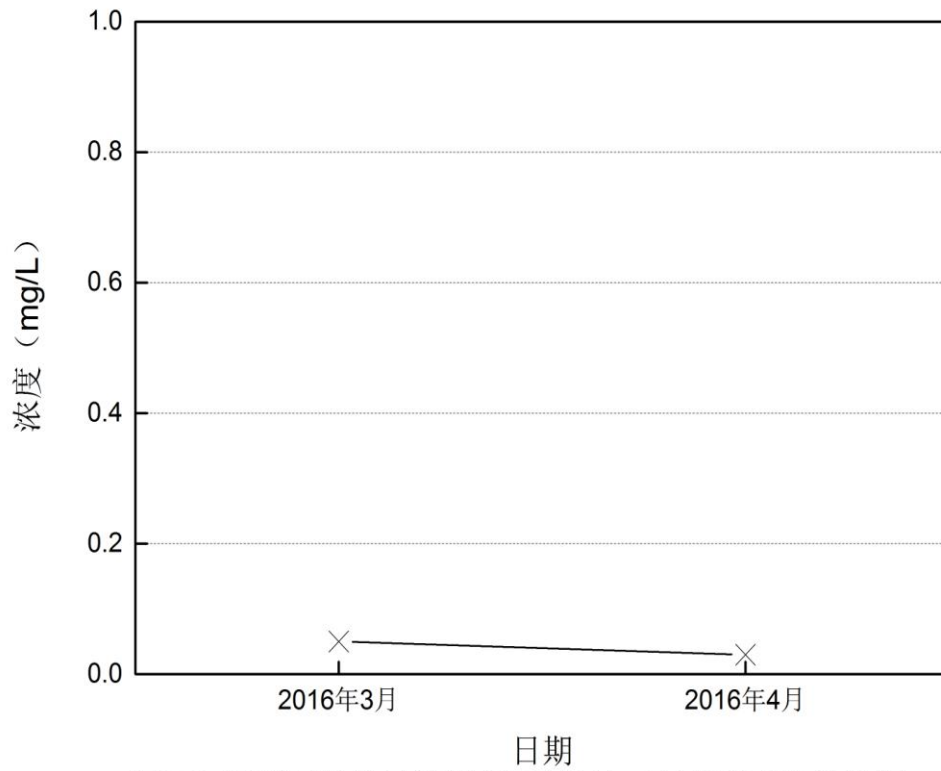
图5-8 深圳河长岭村监测点16年3月~4月总磷变化趋势图
