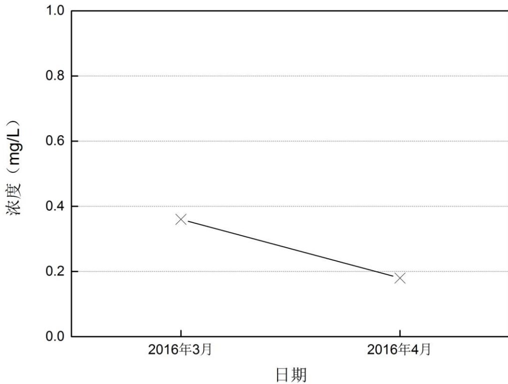
图5-14 深圳河砂石传送带监测点16年3月~4月总磷变化趋势图
