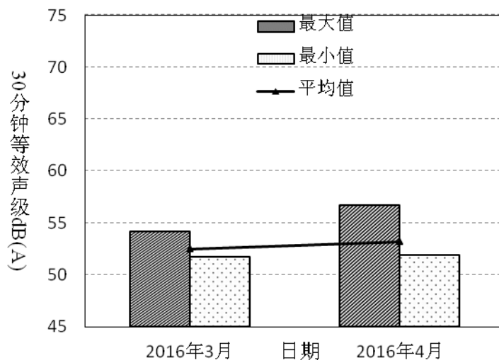
图4-20 香港较寮村2016年3月~4月昼间噪音变化趋势
