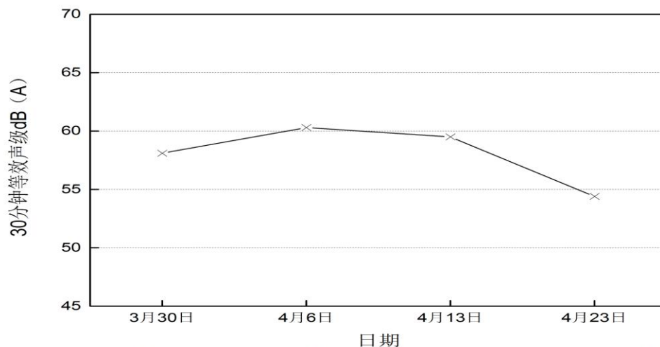
图4-4 2016年4月罗湖区委党校昼夜噪音声级变化趋势
