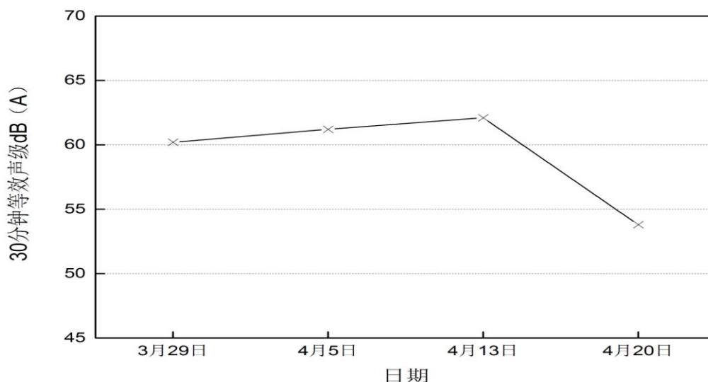
图4-8 2016年4月港莲一村昼夜噪音声级变化趋势
