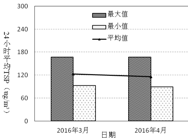
图3-8 2016年3月至4月曦龙山庄24小时TSP变化趋势
