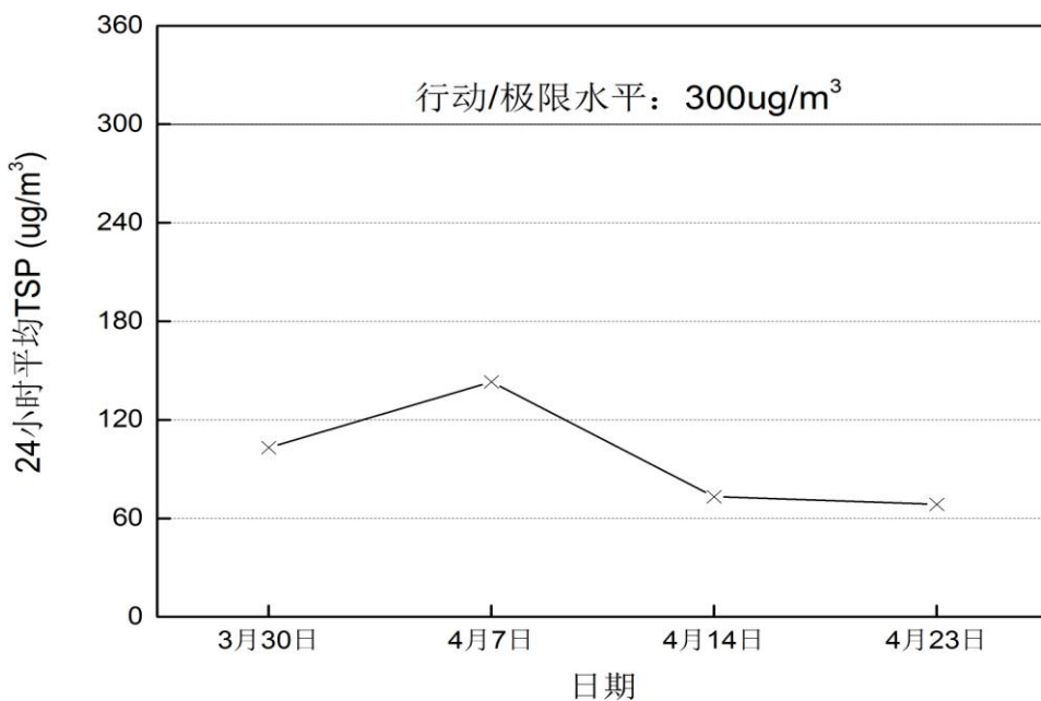
图3-4 2016年4月罗芳村小学和幼儿园24小时平均TSP变化趋势
