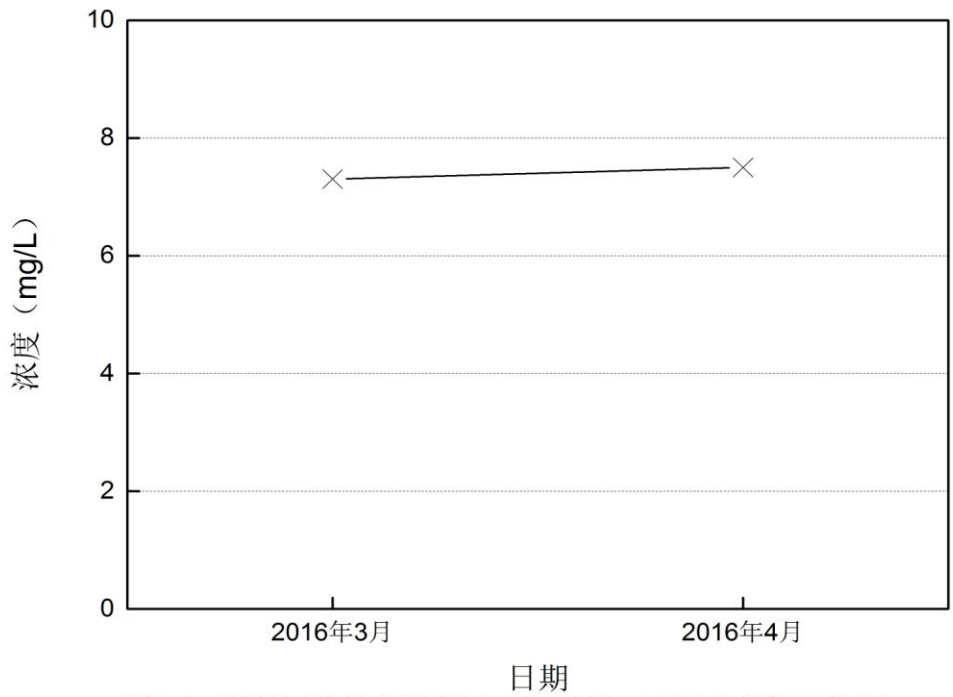
图5-3 深圳河长岭村监测点16年3月~4月DO变化趋势图
