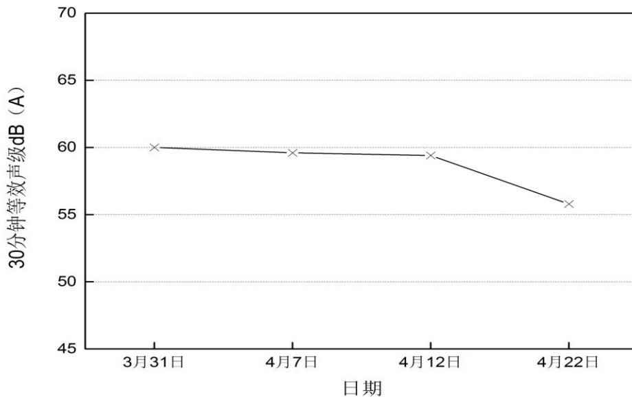
图4-3 2016年4月罗芳村昼夜噪音声级变化趋势
