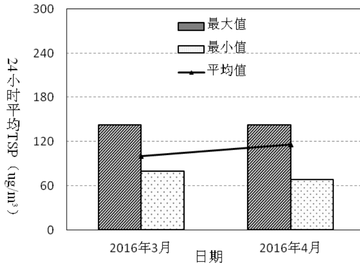
图3-9 2016年3月至4月罗芳村和幼儿园24小时TSP变化趋势
