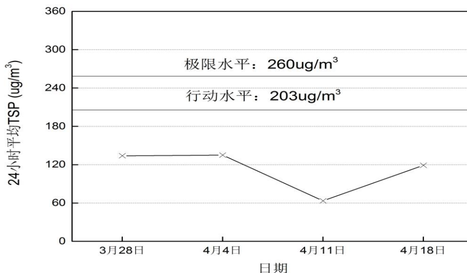
图3-6 2016年4月松园下村24小时平均TSP变化趋势
