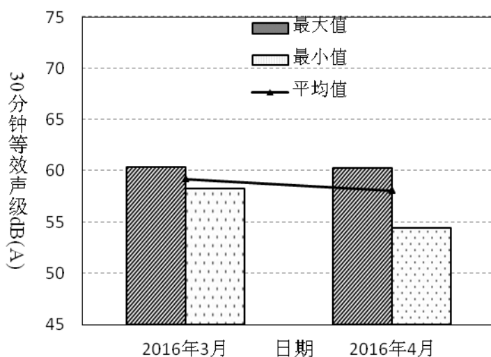
图4-14 罗湖区委党校2016年3月~4月昼间噪音变化趋势
