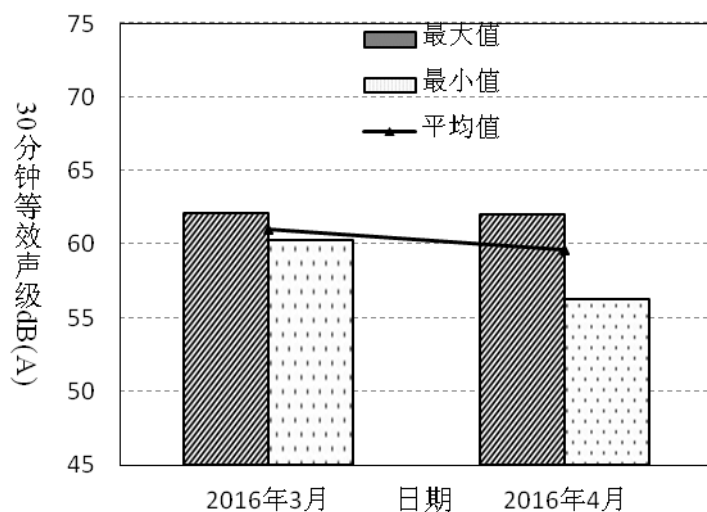
图4-12 罗芳村小学和幼儿园2016年3月~4月昼间噪音变化趋势
