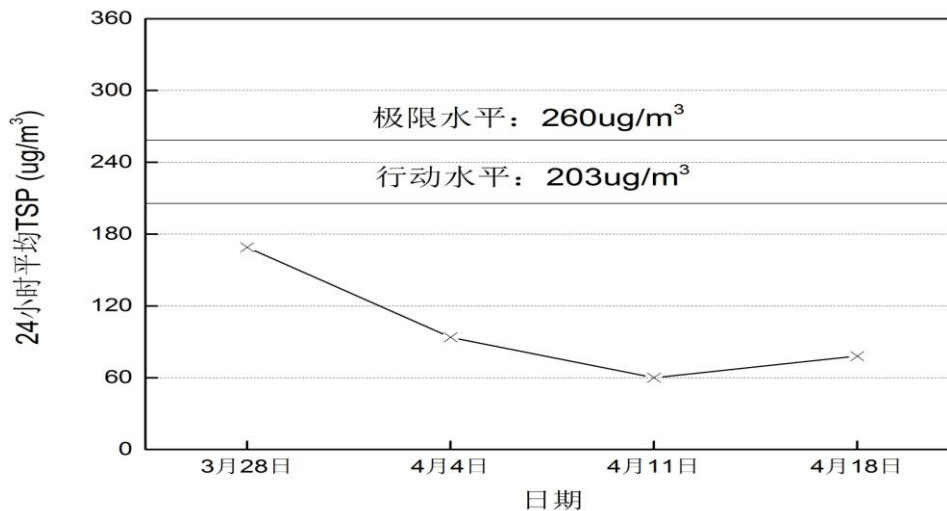
图3-5 2016年4月较寮村24小时平均TSP变化趋势
