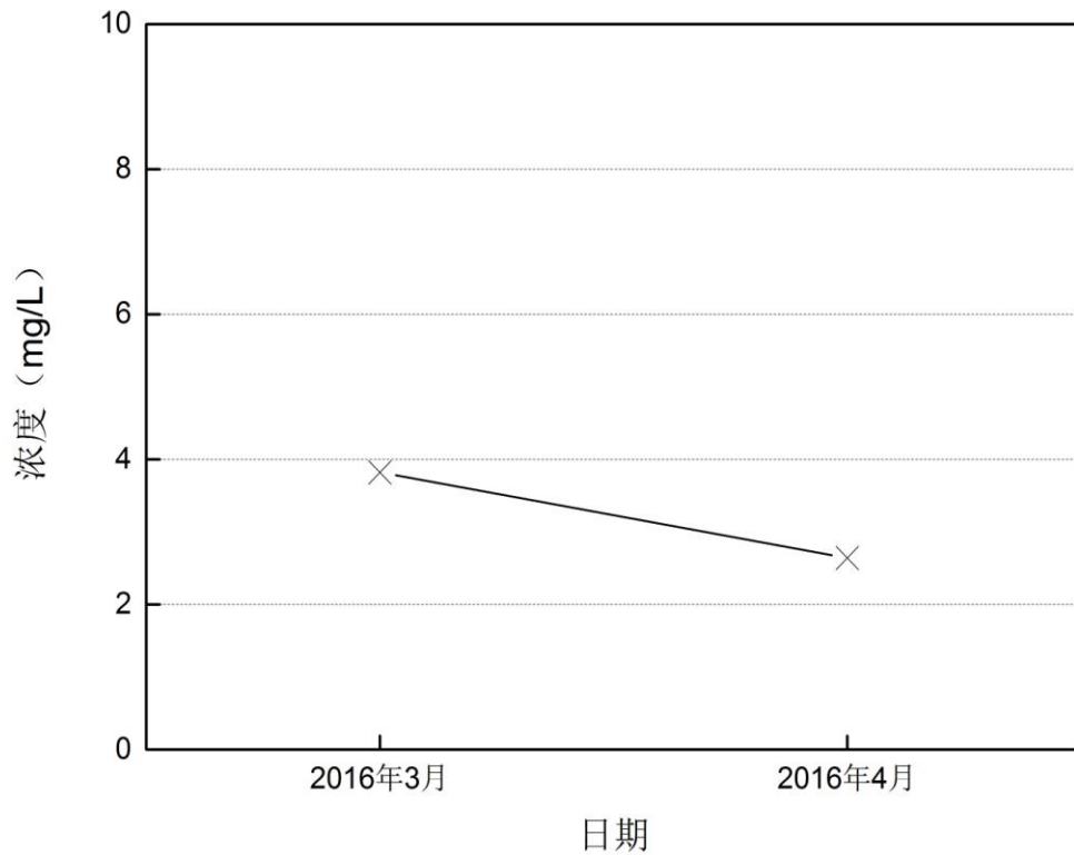
图5-12 深圳河砂石传送带监测点16年3月~4月氨氮变化趋势图
