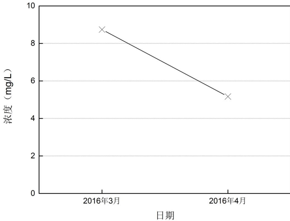
图5-13 深圳河砂石传送带监测点16年3月~4月总氮变化趋势图
