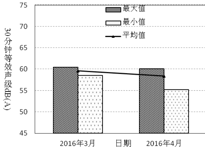
图4-17 鹏兴花园2016年3月~4月昼间噪音变化趋势
