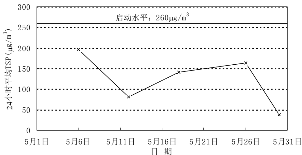
图3-2 2006年5月华侨新村监察点24小时平均TSP变化趋势
