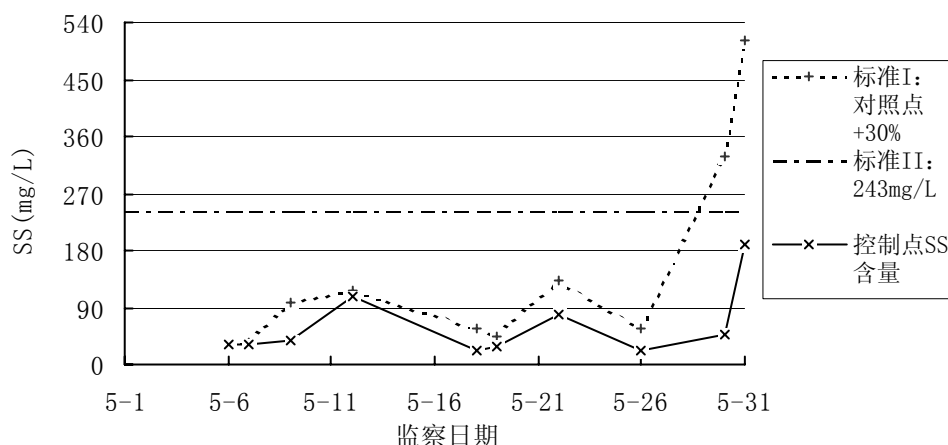
图 5-5 2006 年 05 月 III C 工程落潮期水下疏浚 SS 含量超标情况对照图
