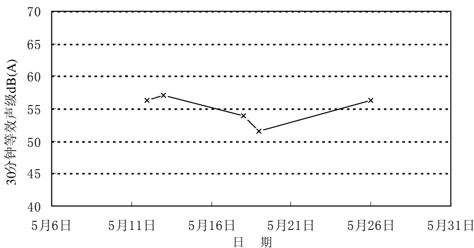
图4-4 2006年5月木湖村监察点昼间噪音声级变化趋势
