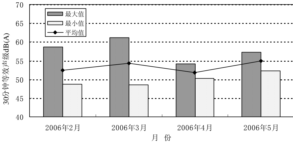
图4-6 2006年2月~5月瓦窑村监察点昼间噪音变化趋势
