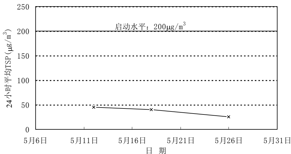
图3-3 2006年5月瓦窑村监察点24小时平均TSP变化趋势
