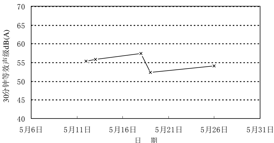
图4-3 2006年5月瓦窑村监察点昼间噪音声级变化趋势
