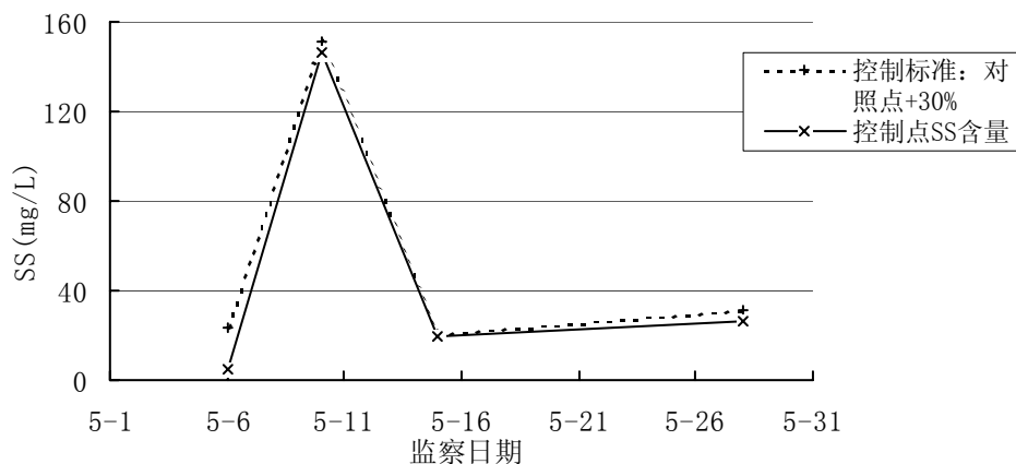
图5-6 2006年05月IIIC工程转运场涨潮期水质监察SS含量超标情况对照图
