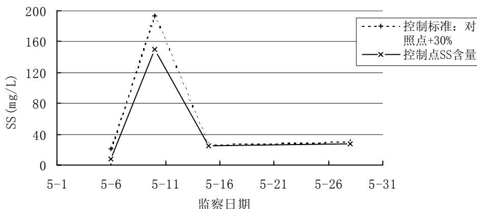
图5-7 2006年05月III C工程转运场落潮期水质监察SS含量超标情况对照图
