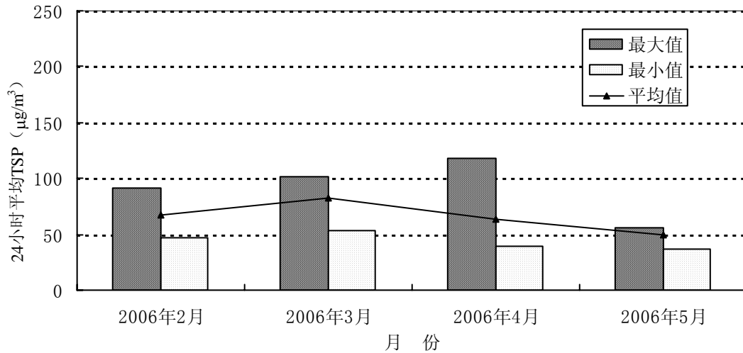
图3-7 2006年2月至5月香港木湖村监察点24小时TSP变化趋势
