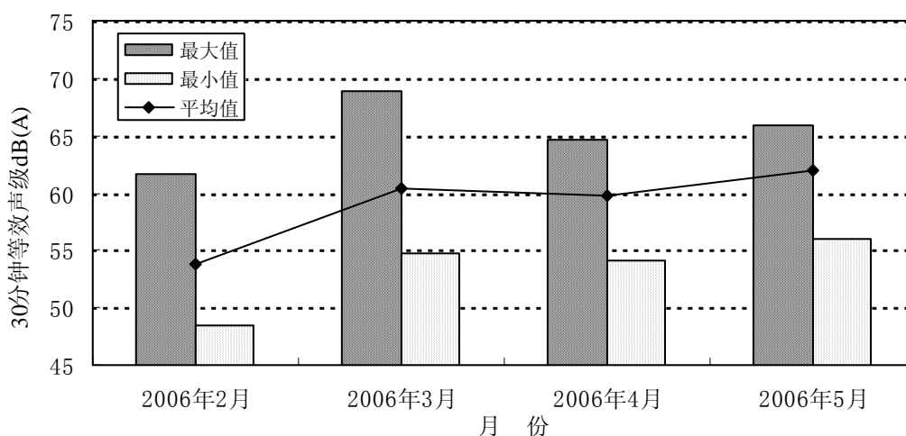
图4-5 2006年2月~5月华侨新村监察点昼间噪音变化趋势
