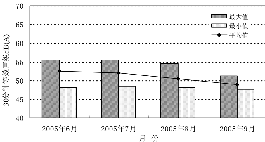
图4-7 香港木湖村05年06月~09月昼间噪音变化趋势
