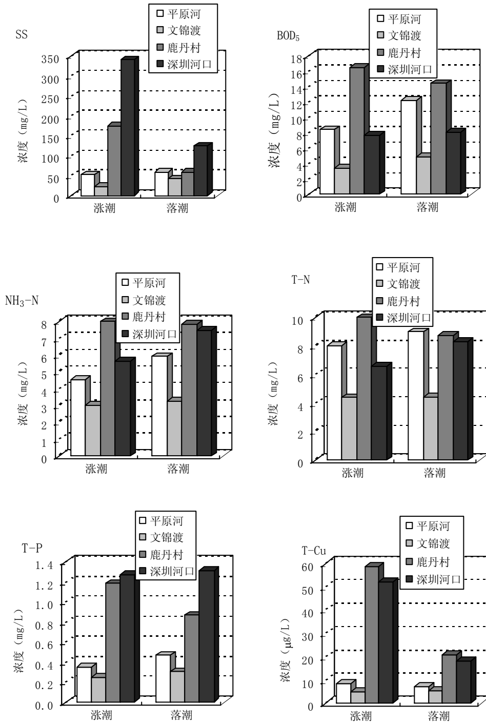
图 5-2 2005 年 9 月 21 日深圳河水质沿程变化图
