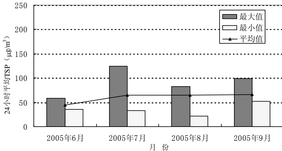
图3-6 05年06月至09月香港瓦窑村24小时TSP变化趋势
