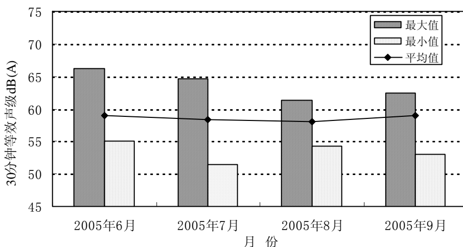
图4-5 华侨新村05年06月~09月昼间噪音变化趋势
