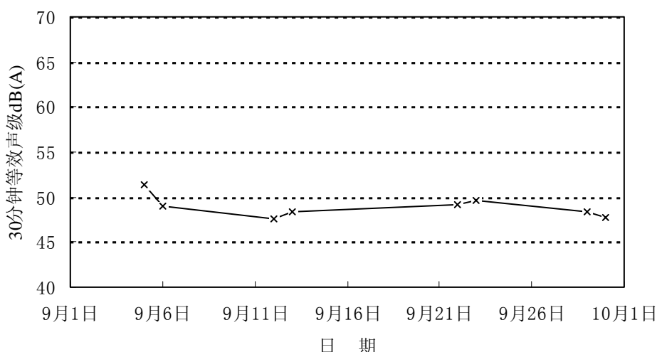
图4-4 2005年9月木湖村昼间噪音声级变化趋势
