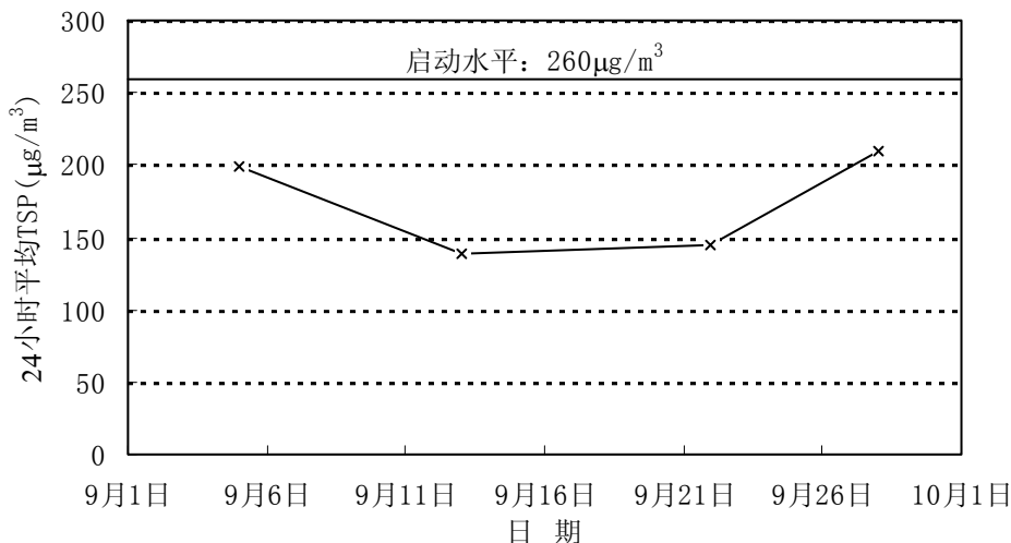
图3-2 2005年9月华侨新村24小时平均TSP变化趋势
