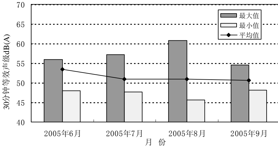
图4-6 香港瓦窑村05年06月~09月昼间噪音变化趋势
