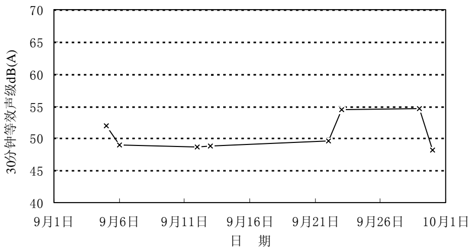
图4-3 2005年9月瓦窑村昼间噪音声级变化趋势
