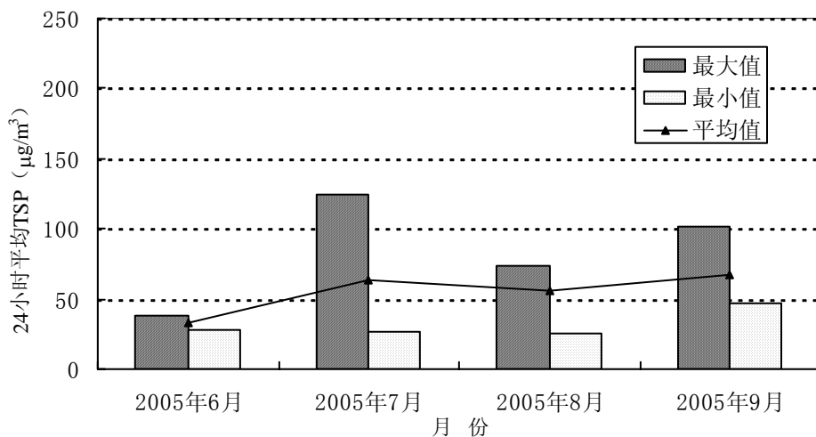
图3-7 05年06月至09月香港木湖村24小时TSP变化趋势
