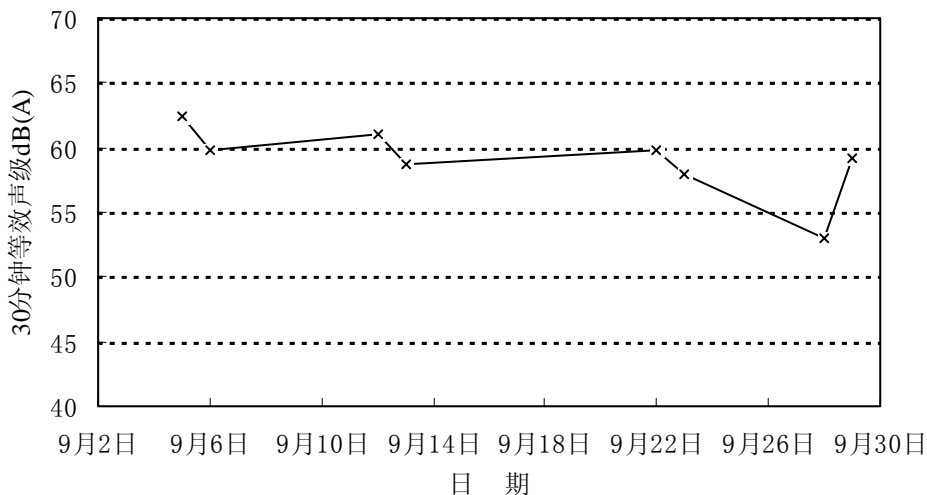
图4-2 2005年9月华侨新村昼间噪音声级变化趋势
