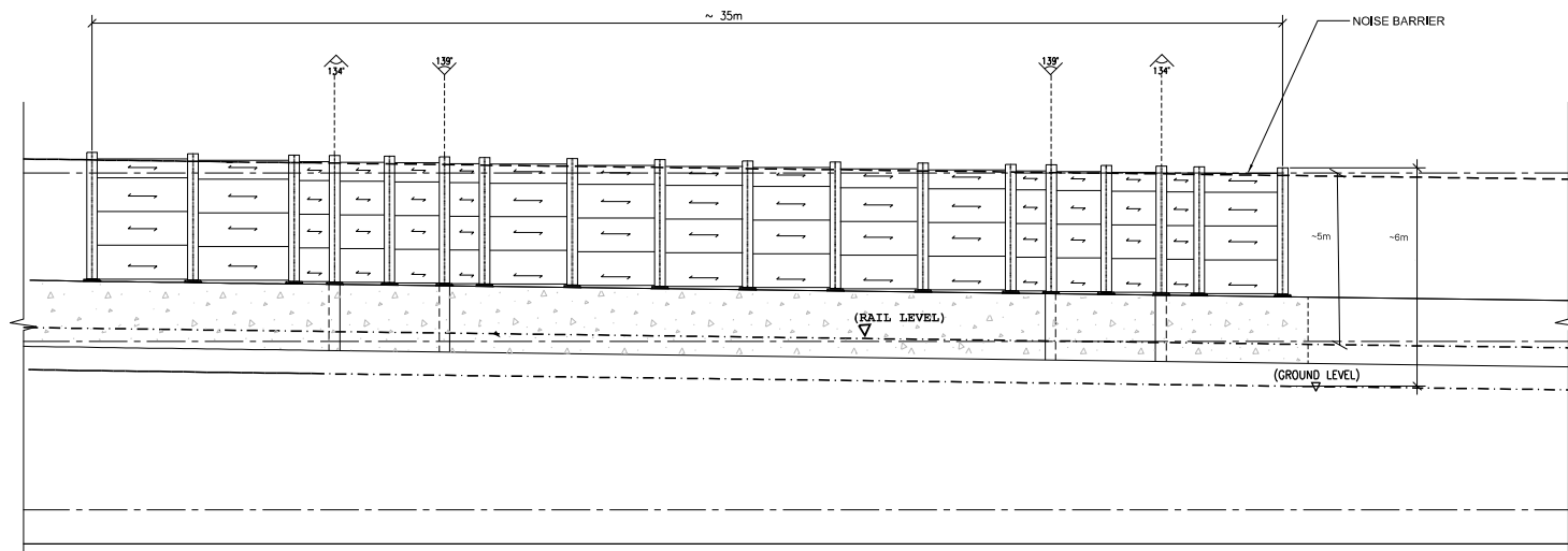
ELEVATION B 002
