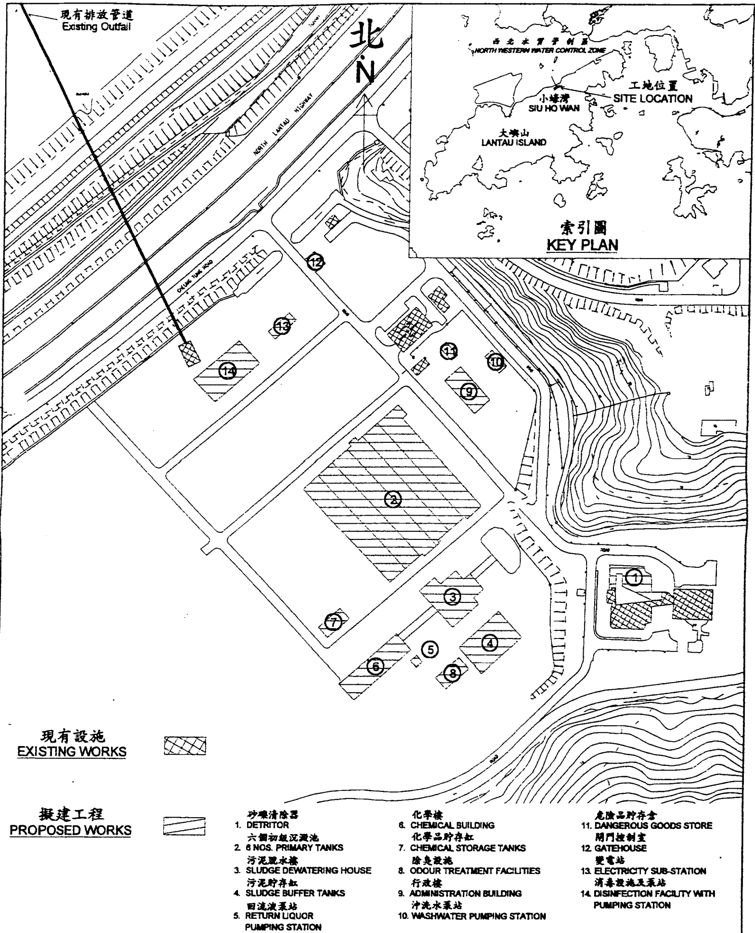
Figure 1 圖一 小墟灣污水處理廠改善工程 UPGRADING OF SIU HO WAN SEWAGE TREATMENT PLANT
