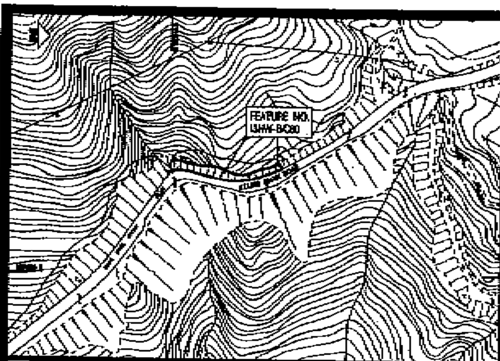
LOCATION PLAN 平面定位圖 SCALE 1:500
