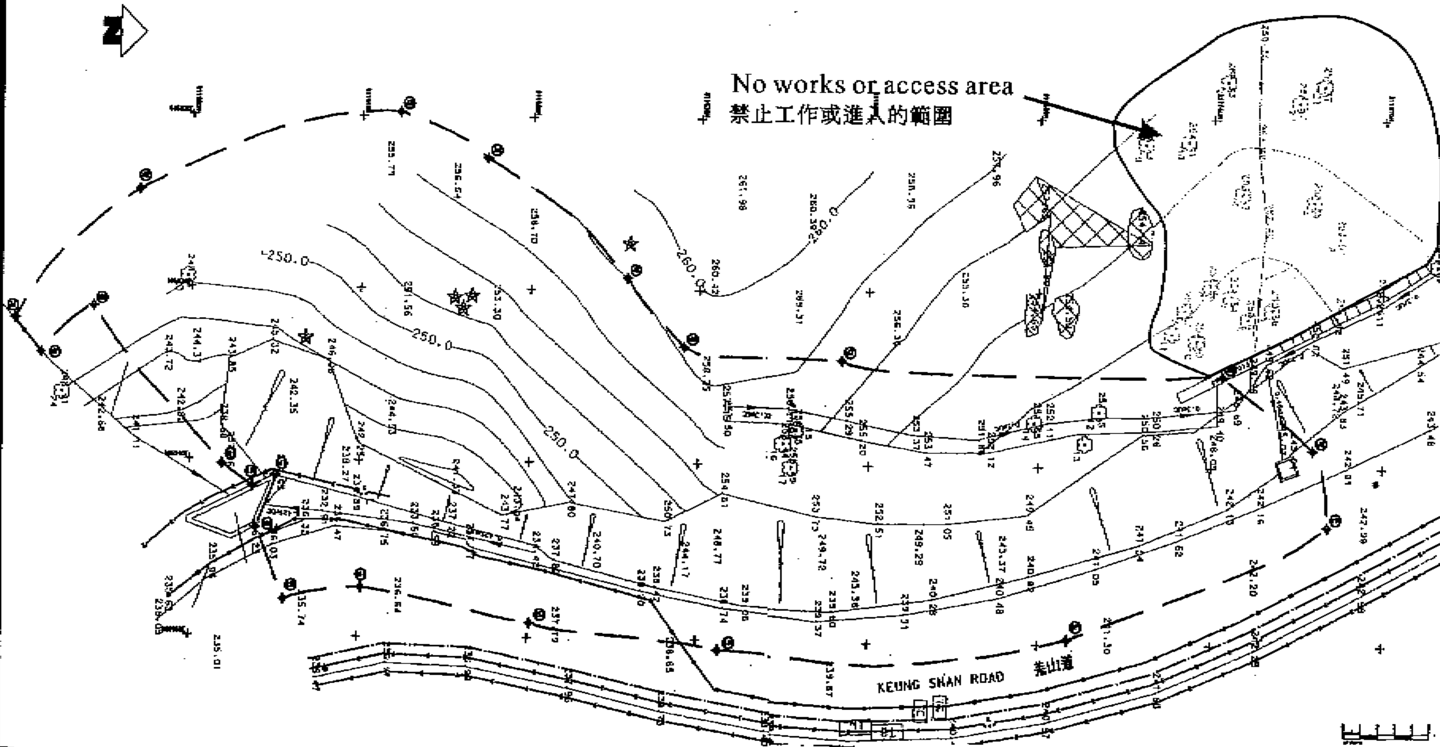
Figure 3 No Works or Access Area at Slope No.13NW-B/C80 圖 3 斜坡編號13NW-B/C80禁止工作或進入的範圍
