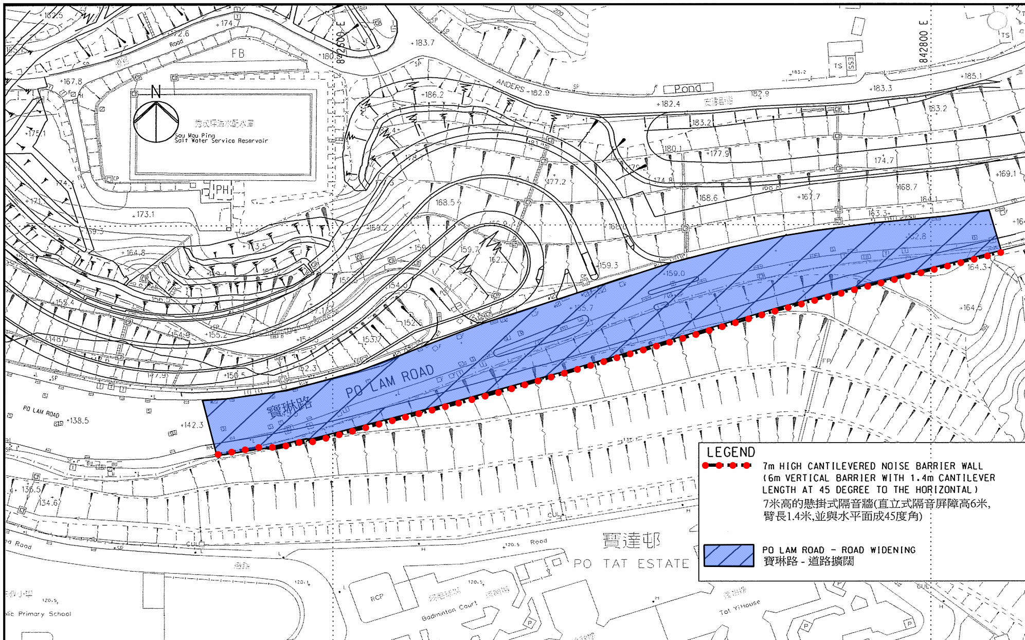
Figure 1: Po Lam Road – Road Widening 圖 1 : 寶琳路 – 道路擴闊工程
