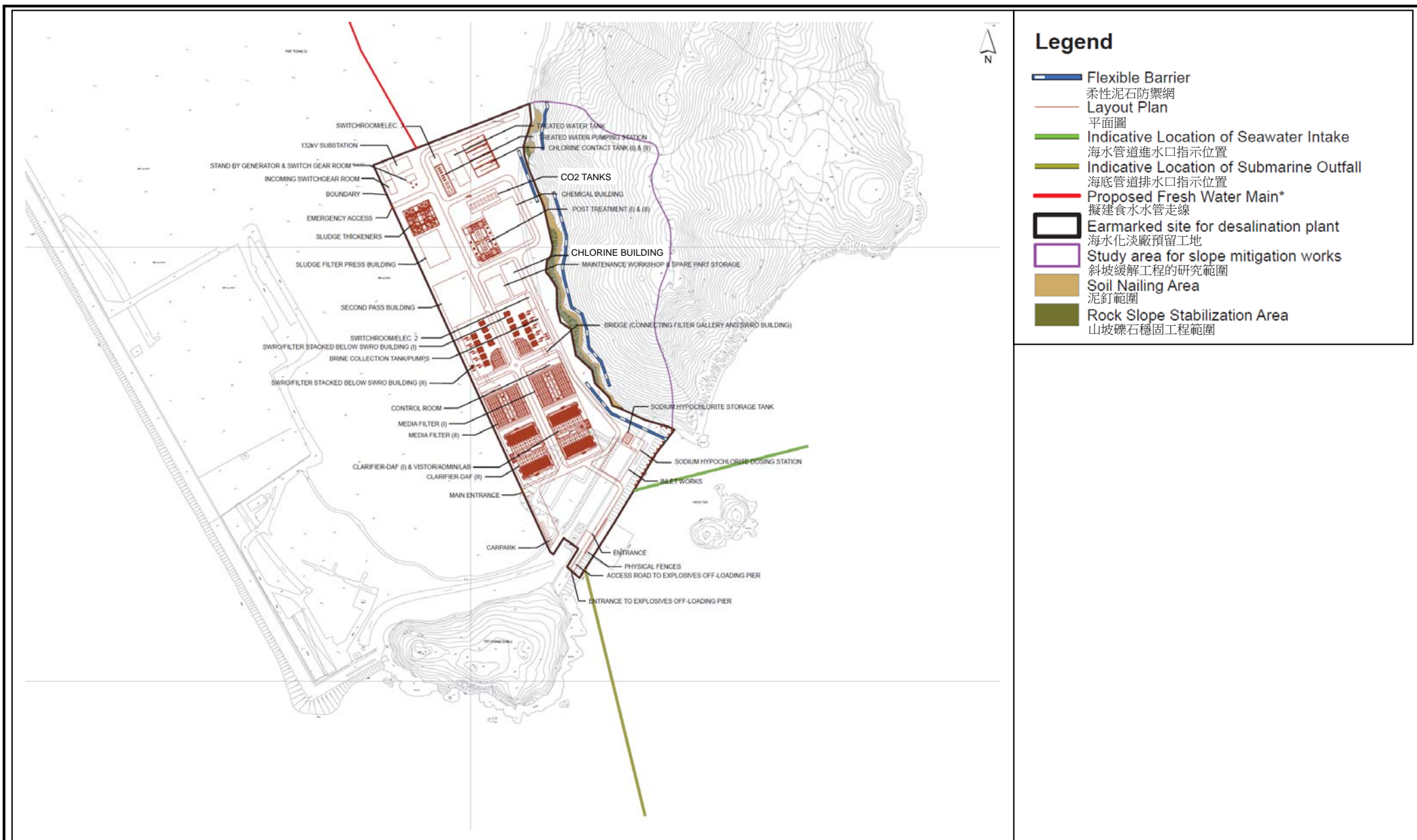
Project Title: Desalination Plant at Tseung Kwan O 工程項目名稱：將軍澳海水化淡廠 Layout Plan of the Project 工程項目平面圖
