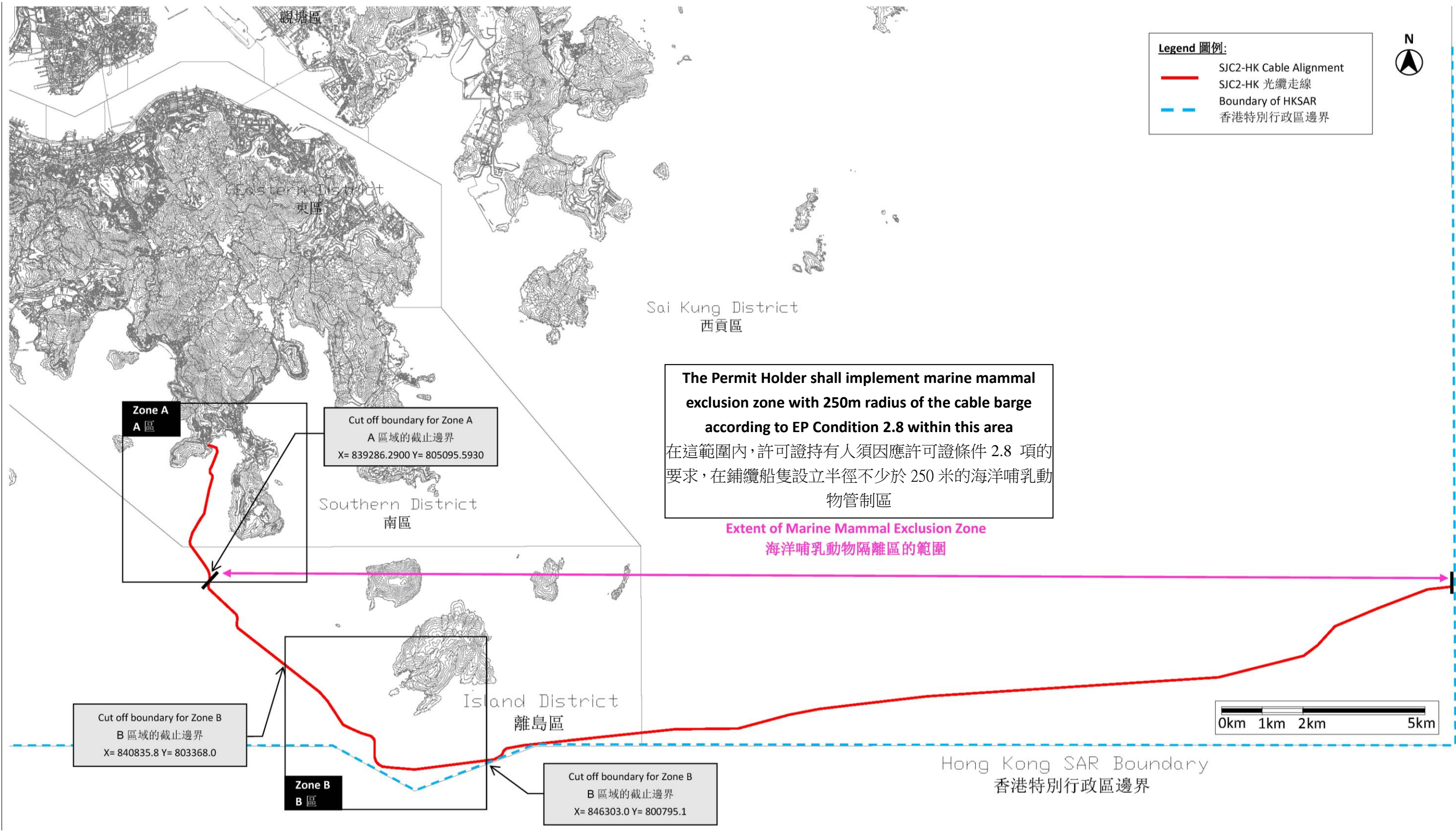
Project Title 工程項目名稱 South East Asia - Japan 2 Cable System - Hong Kong Segment (SJC2-HK) - Chung Hom Kok 東南亞 - 日本二號光纜系統 - 香港段(SJC2-HK) - 春坎角 Figure 4 圖 4 Cable Installation / Repair Works Area Where Marine Mammal Exclusion Zone Shall Be Implemented 須要設置海洋哺乳動物管制區的海底光纜鋪設工程/維修工程範圍
