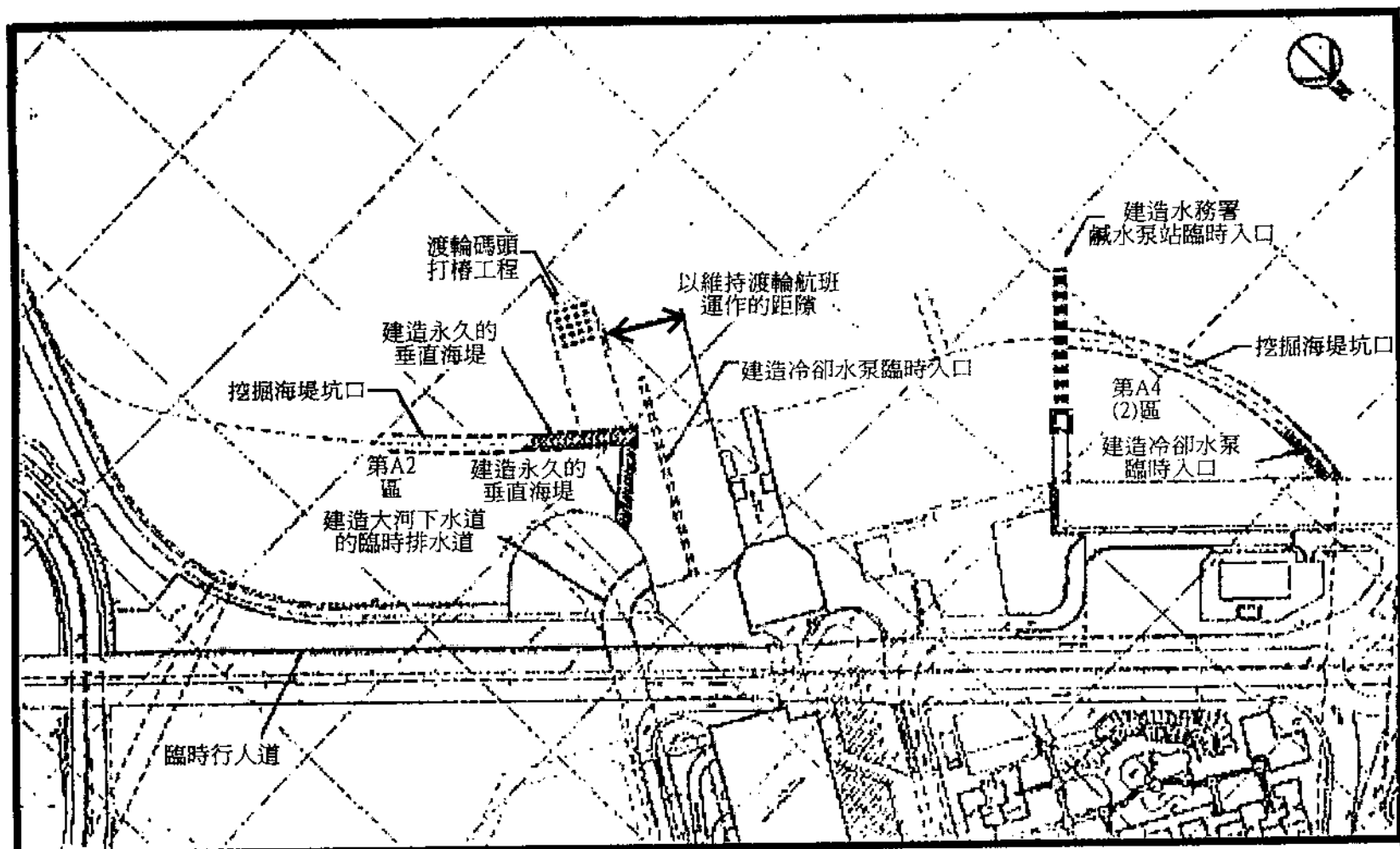
圖1 — 第一期荃灣海灣填海工程
