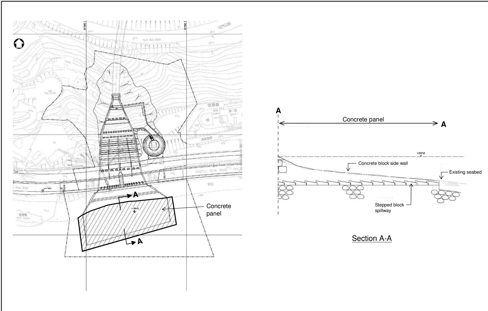
Figure 8 : Outfall 圖 8: 出水口
