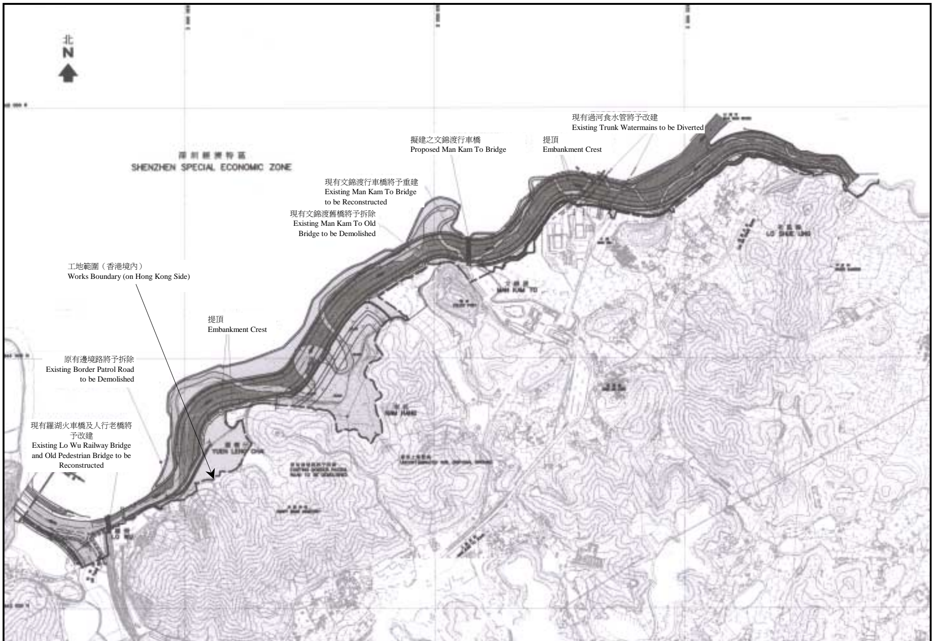
圖 1 治理深圳河第三期工程 — 位置圖 Figure 1 Shenzhen River Regulation Project Stage III — Site Plan
