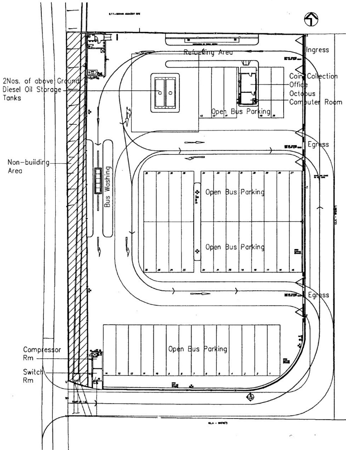
Figure 2 : Layout Plan of the Proposed Temporary Bus Depot at Tseung Kwan O, Area 85 圖2: 建議中的將軍澳85區的臨時巴士車廠設計圖
