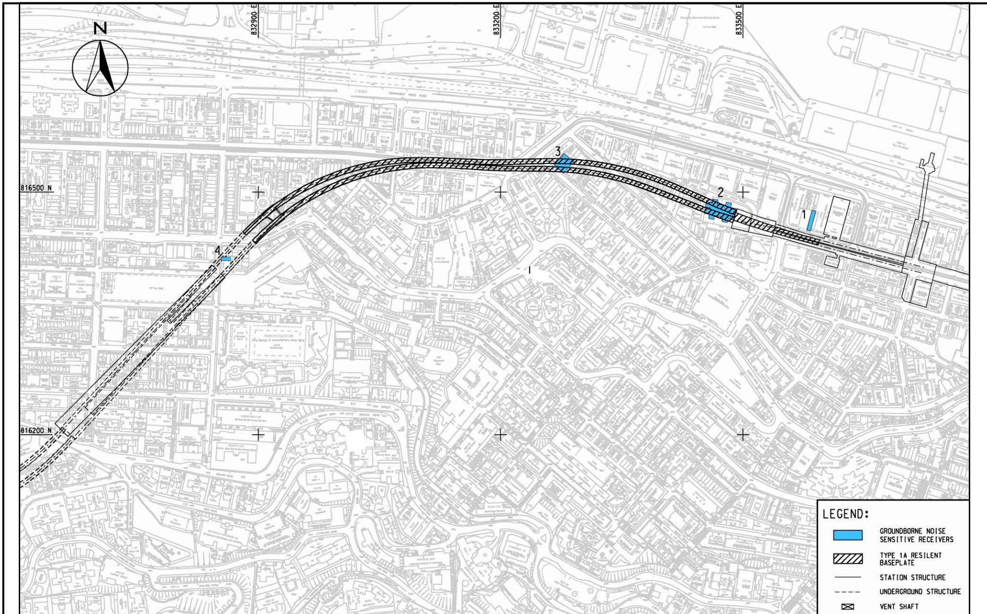
Figure 17: Rail Track Type 圖 17: 列車路軌類形
