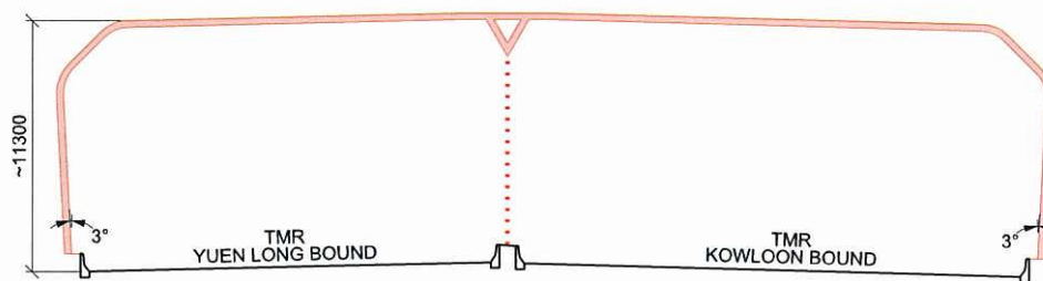
SECTION 13-13 FULL ENCLOSURE NM 19 (N.T.S.)
