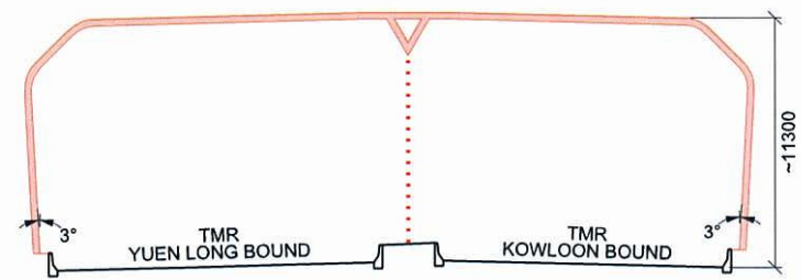
SECTION 12-12 FULL ENCLOSURE NM 19 (N.T.S.)
