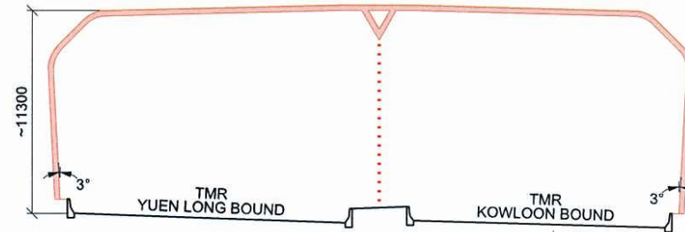
SECTION 4-4 FULL ENCLOSURE NM 8 (N.T.S.)
