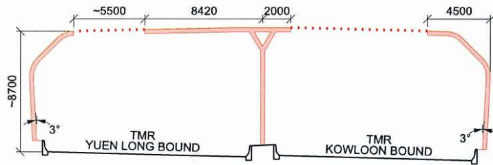
SECTION 3-3 SEMI-ENCLOSURE NM 4 (N.T.S.)
