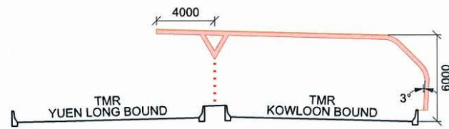
SECTION 6-6 SEMI-ENCLOSURE NM 11 (N.T.S.)
