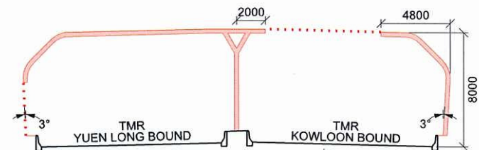
SECTION 8-8 SEMI-ENCLOSURE NM 15 (N.T.S.)
