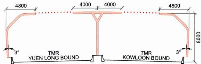
SECTION 7-7 SEMI-ENCLOSURE NM 12 (N.T.S.)
