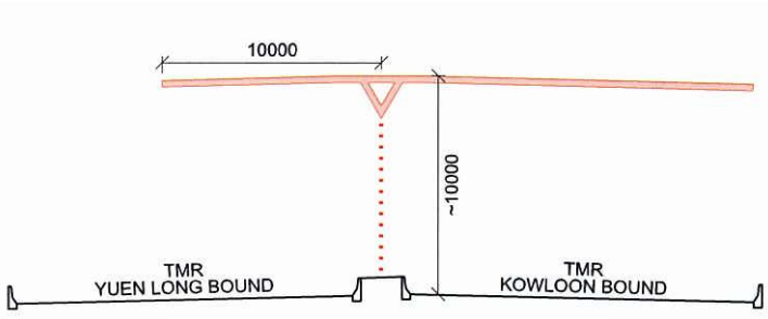
SECTION 10-10 SEMI-ENCLOSURE NM 17 (N.T.S.)
