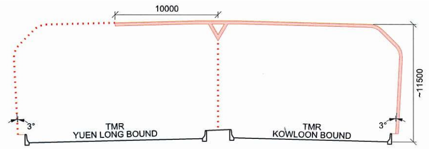
SECTION 11-11 SEMI-ENCLOSURE NM 18 (N.T.S.)
