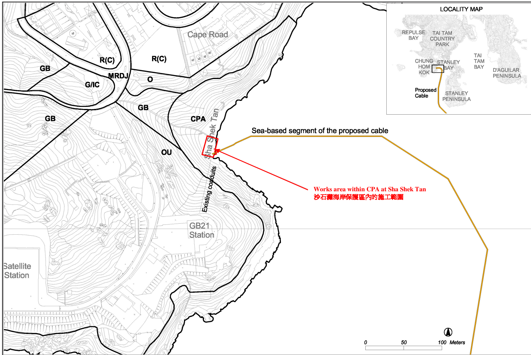
Figure 4: Location Plan of the Works Area at Sha Shek Tan 圖 4: 沙石灘施工範圍的位置圖
