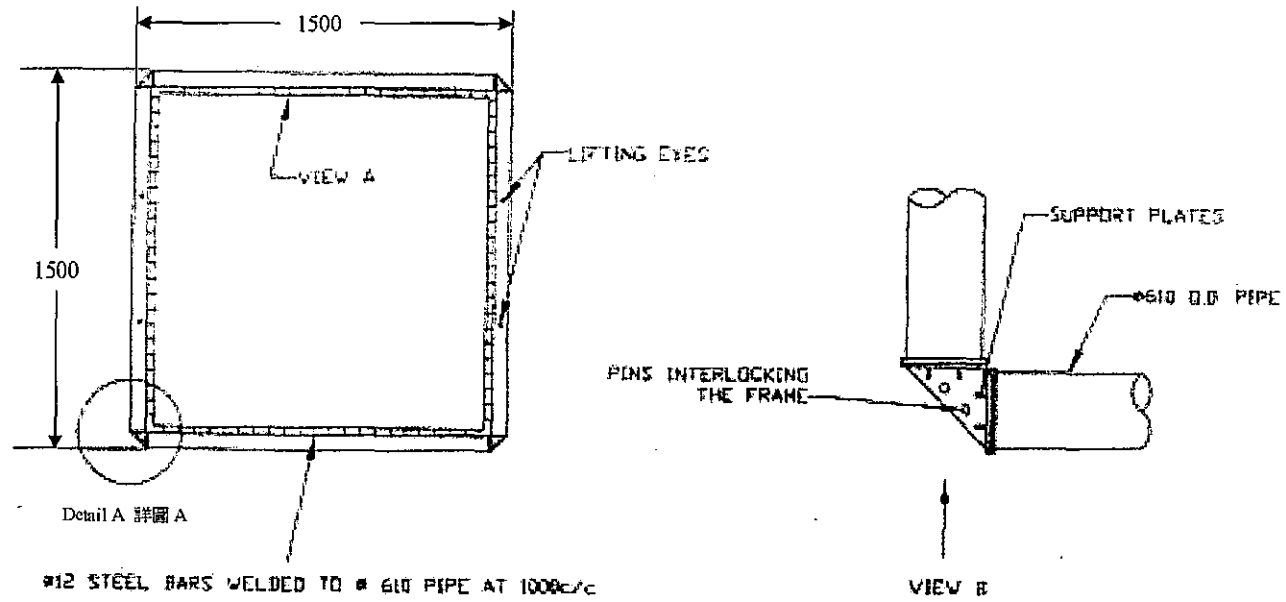
Detail A 詳圖 A
