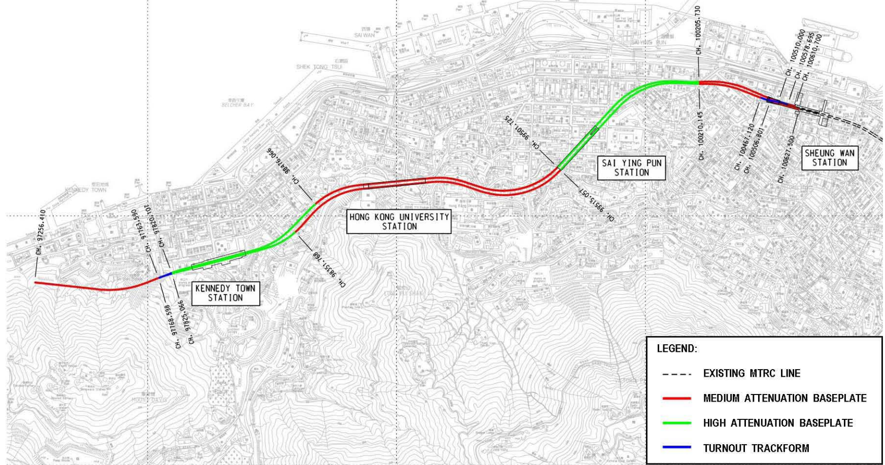
Figure 18: Rail Track Type 圖 18: 列車路軌類形
