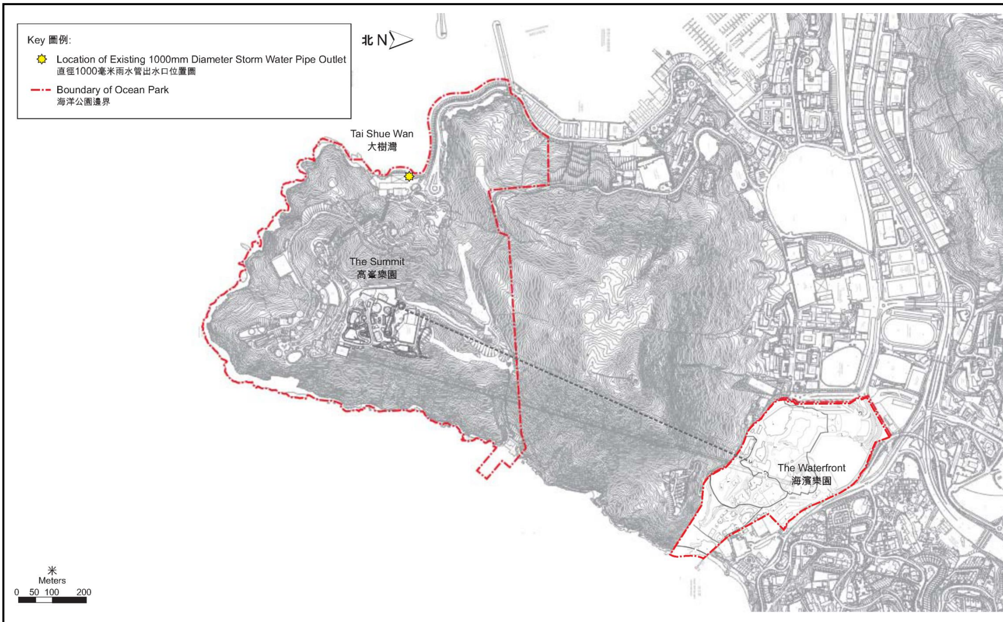
Figure 3: Location of Existing 1000mm Diameter Storm Water Pipe Outlet at Tai Shue Wan 圖 3 : 大樹灣現有直徑 1 000 毫米雨水管出水口位置圖
