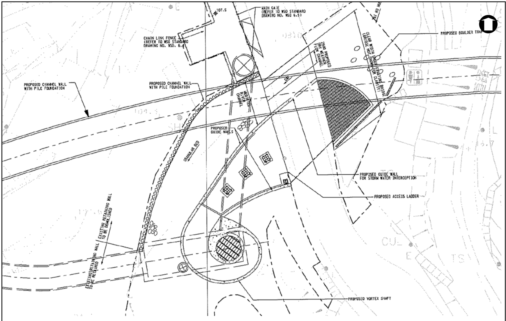
Figure 2 : Works of Intake I-2 at Sam Dip Tam Stream 圖 2: 位於三疊潭河道的收水口I-2工程圖
