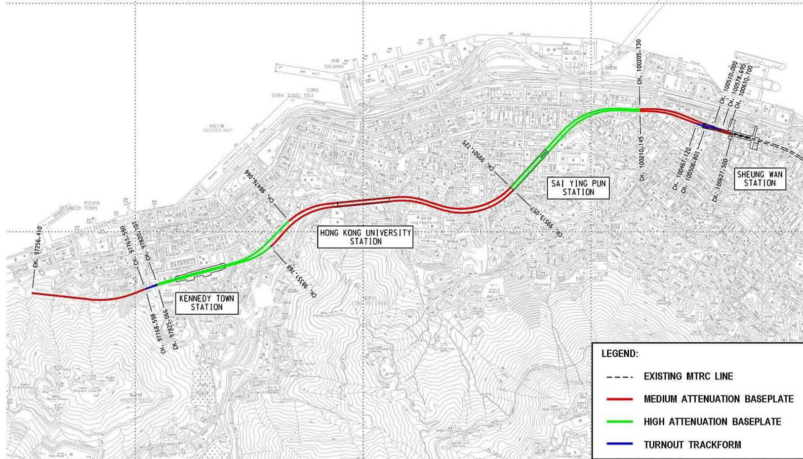
Figure 16: Rail Track Type 圖 16: 列車路軌類形
