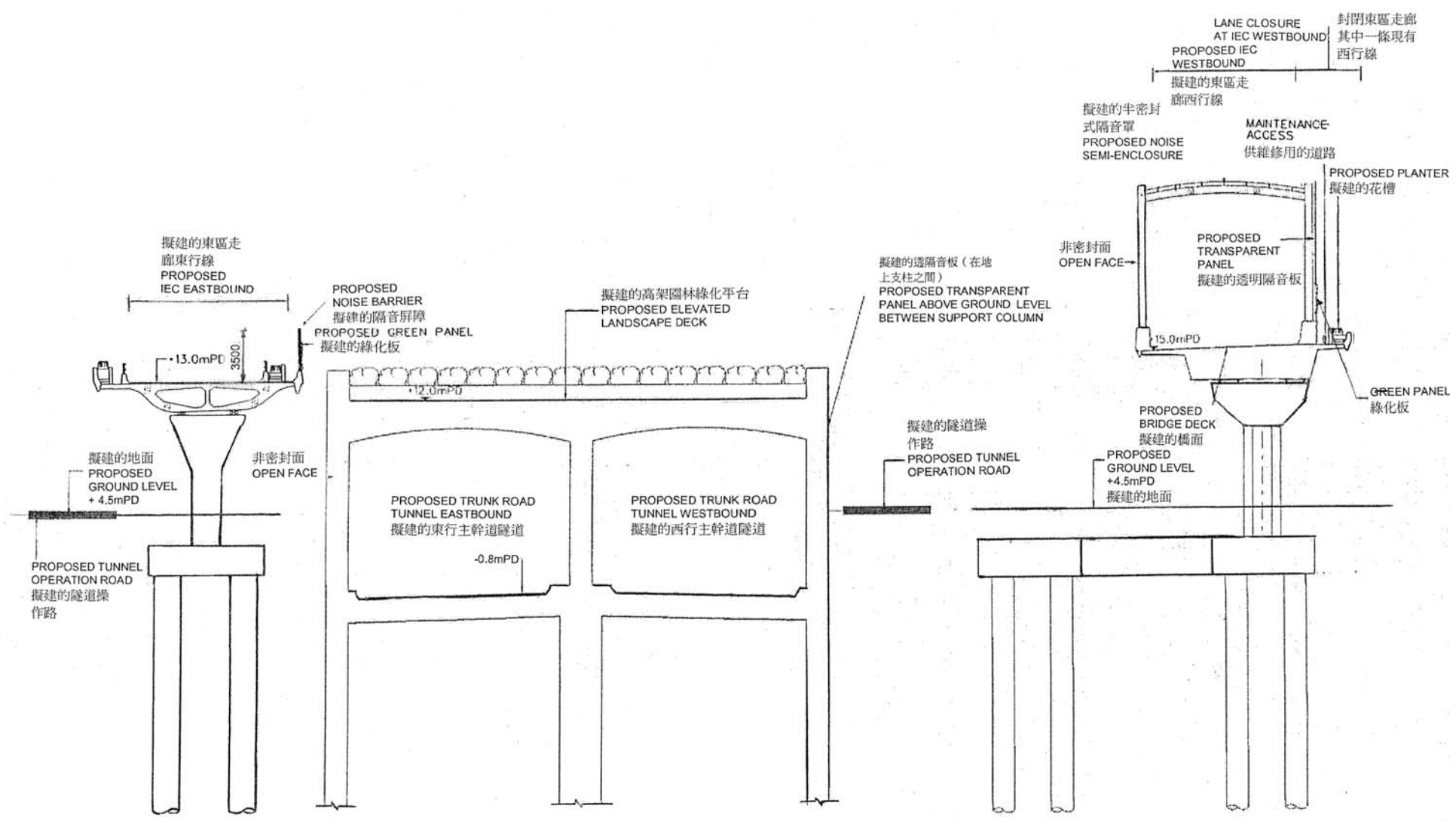
切面 B-B SECTION B-B
