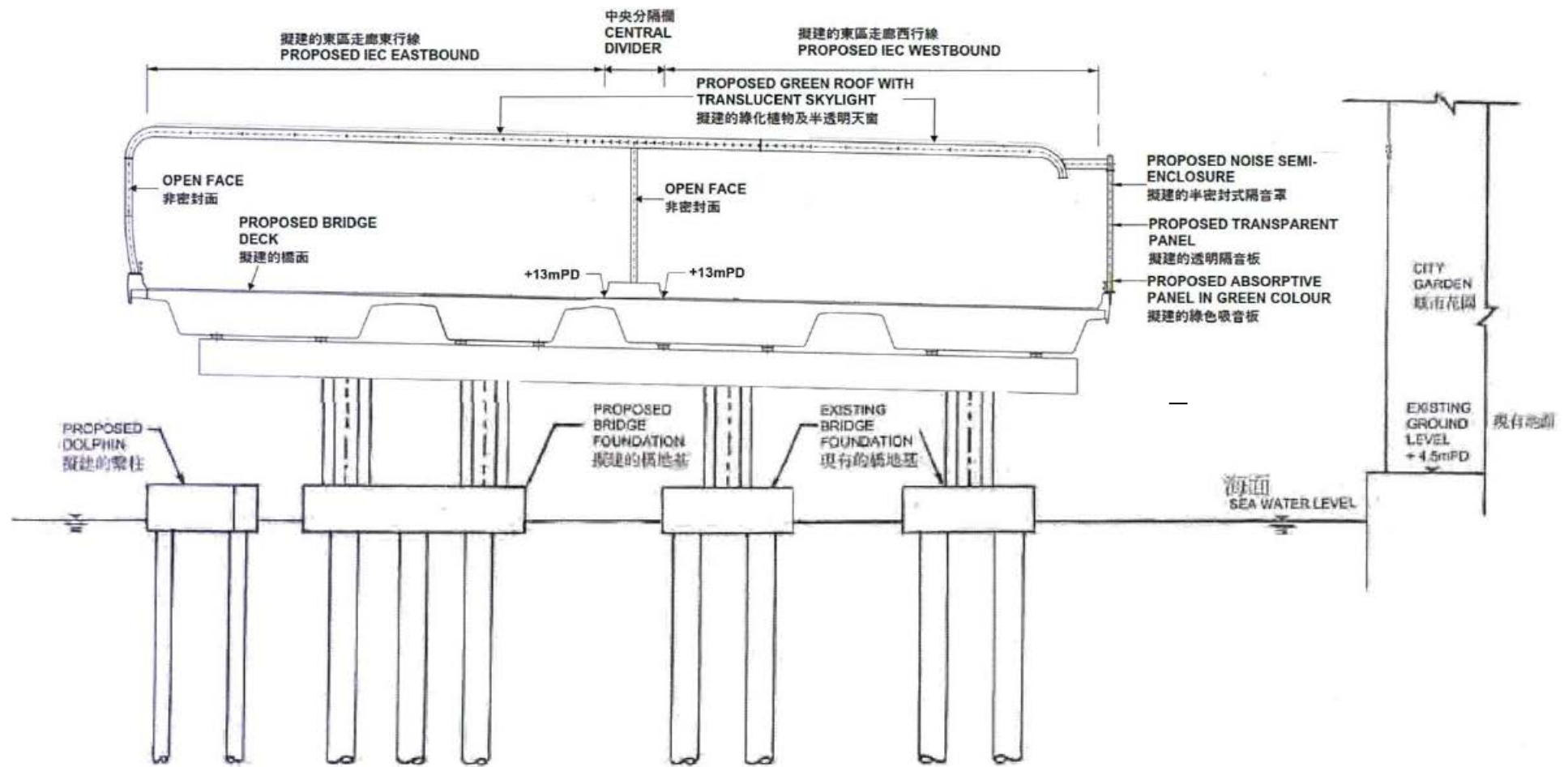
切面 C-C
