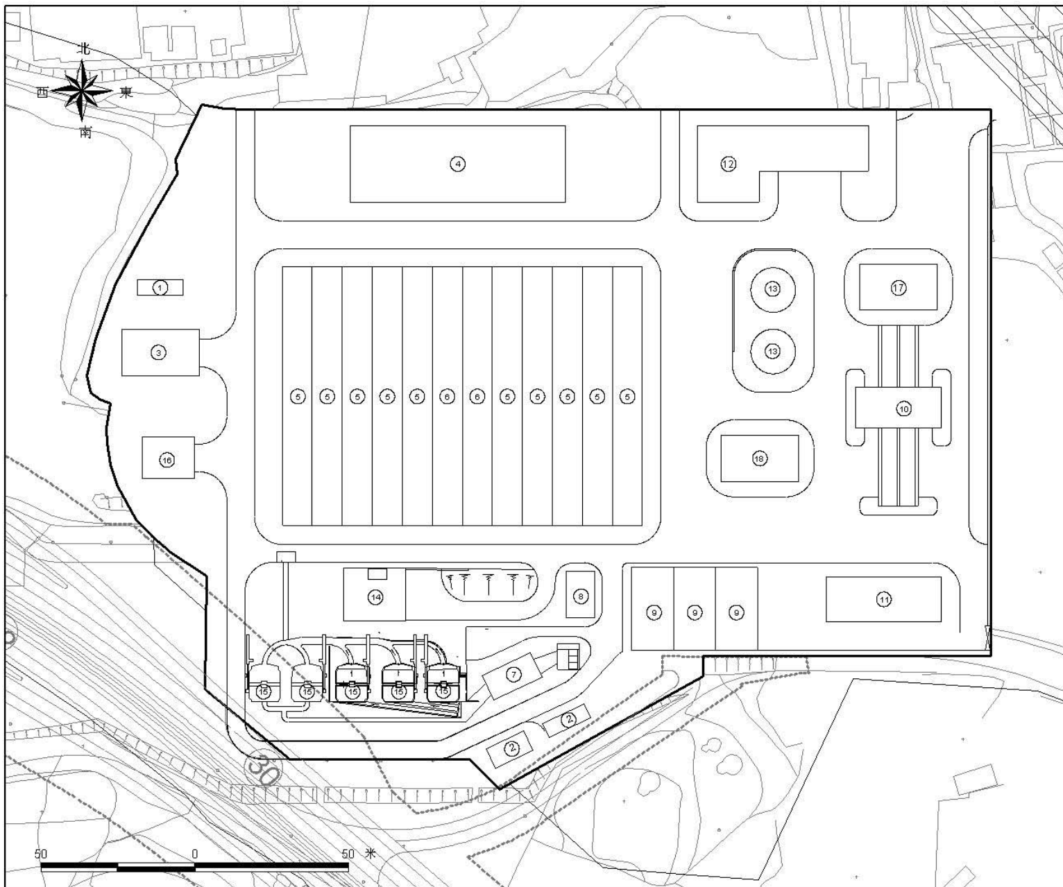
圖四 新圍污水處理廠改善和擴建的規劃佈局圖
