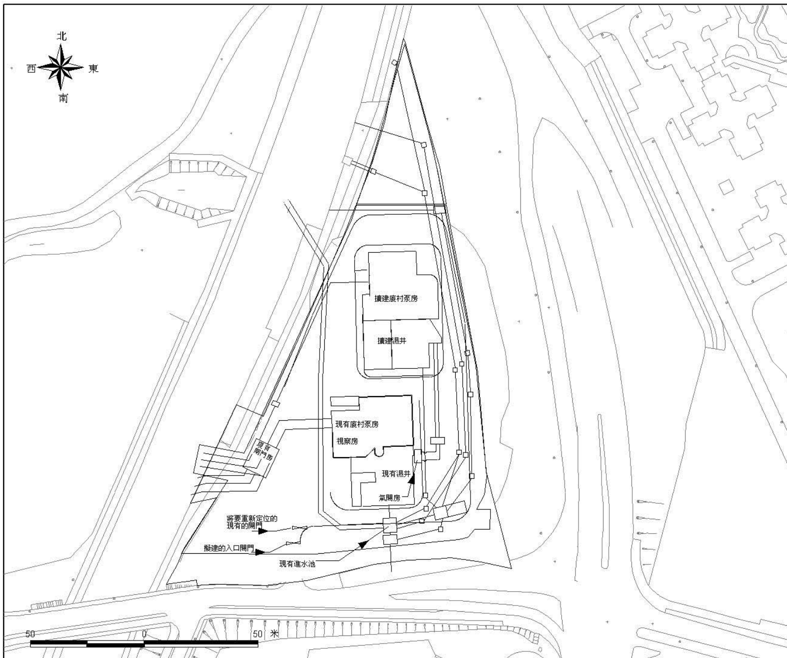
圖五 廢村污水泵站擴建的規劃佈局圖
