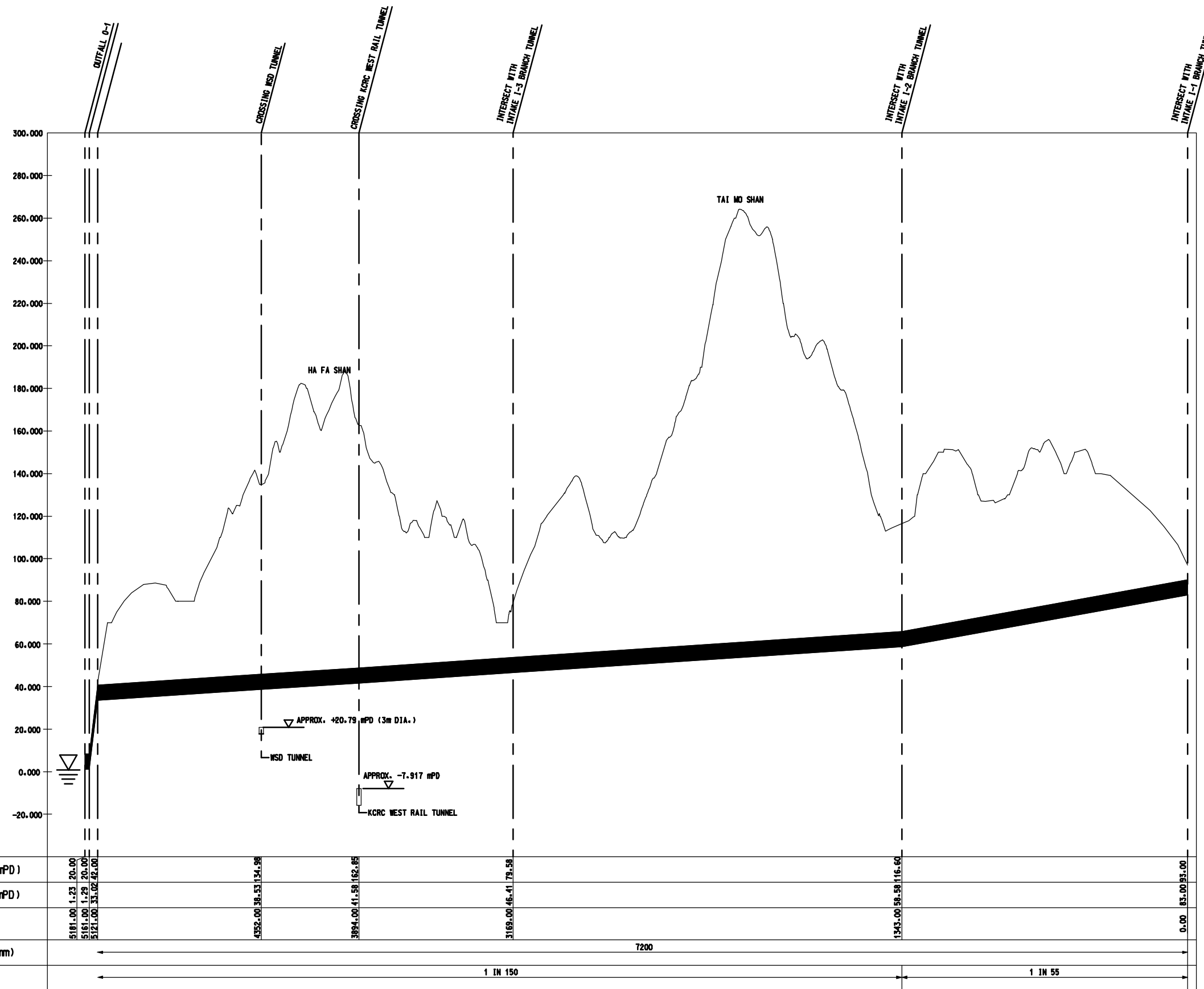
LONGITUDINAL PROFILE
