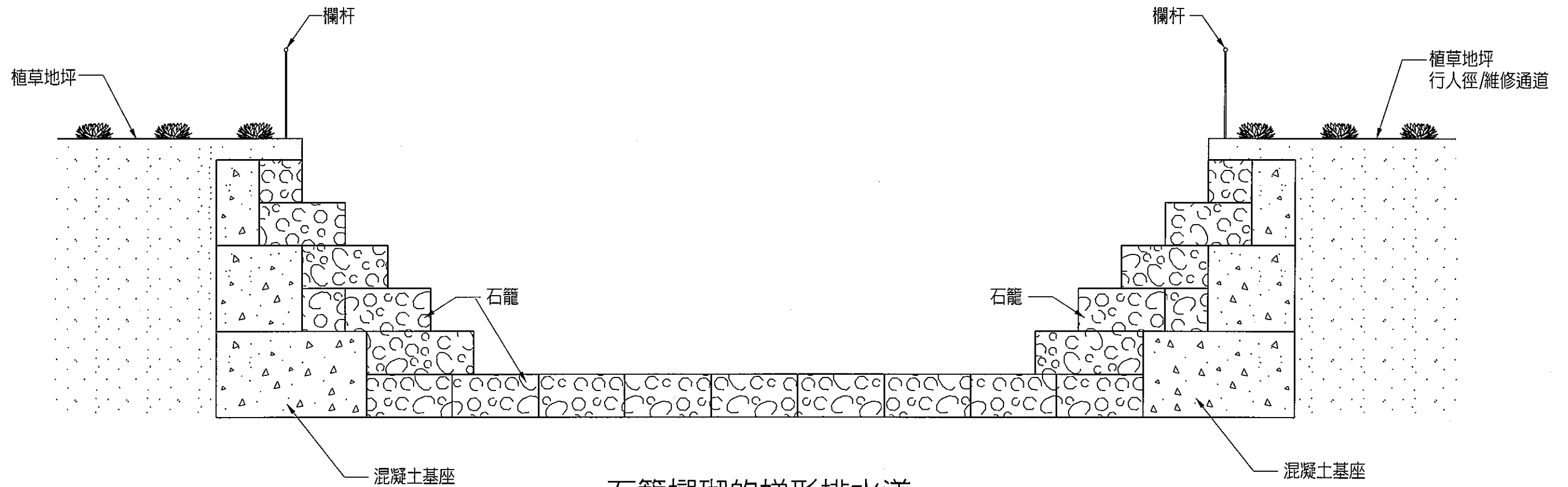
石籠襯砌的梯形排水道
