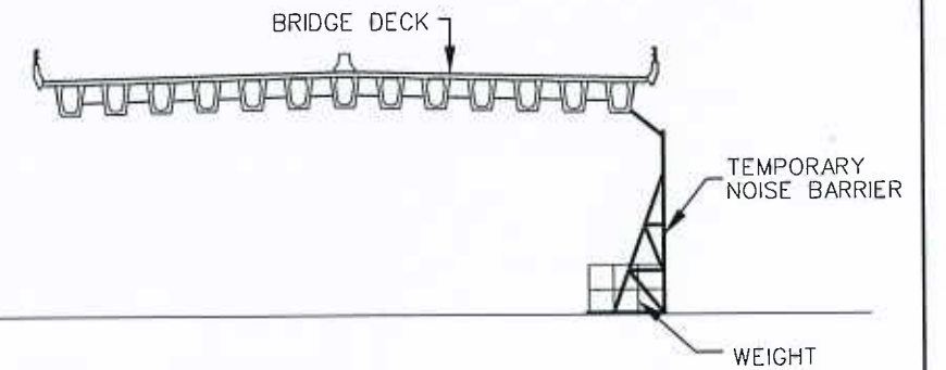
TYPICAL SECTION A-A N.T.S.
