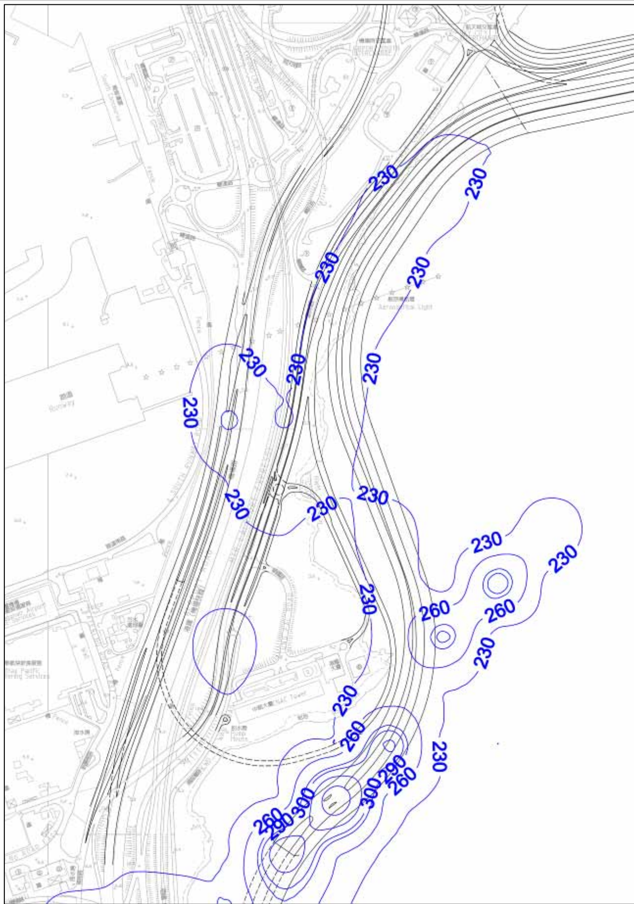
1-hr NO 2
