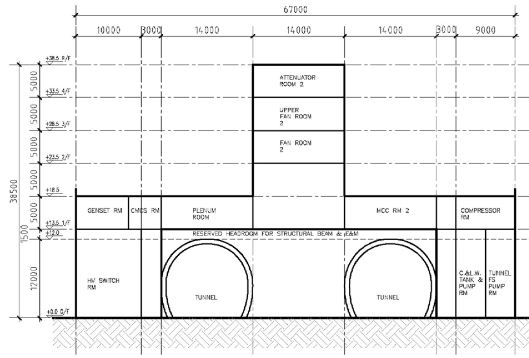
SECTION A-A
