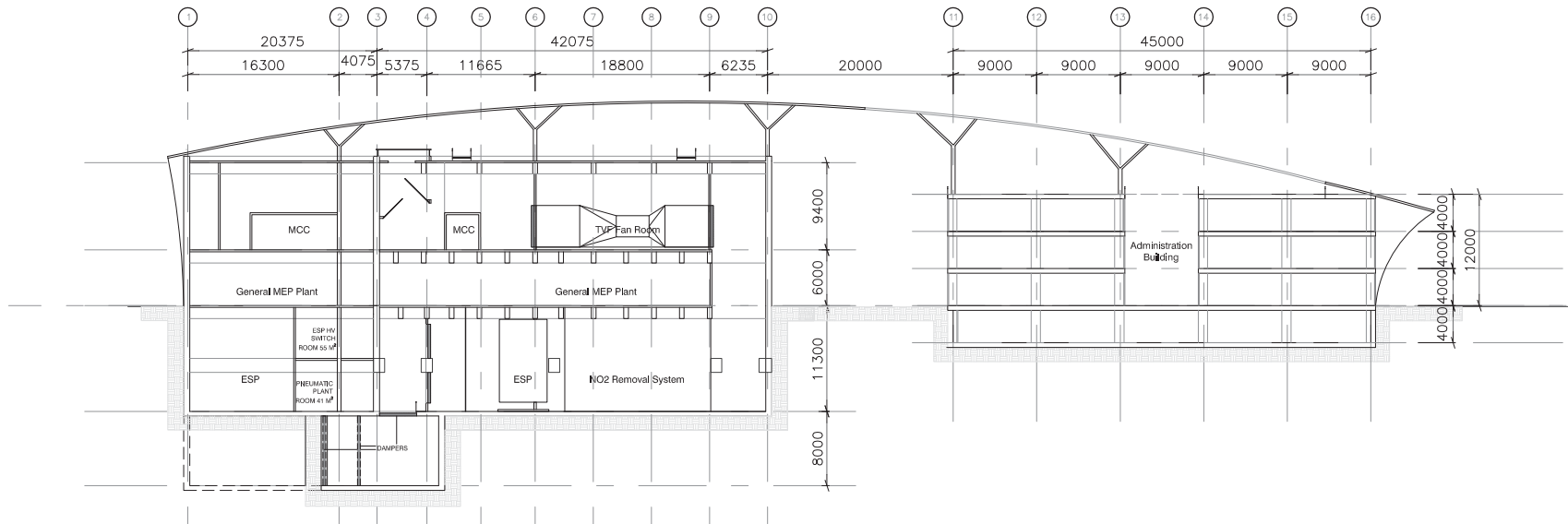
SECTION A-A'
