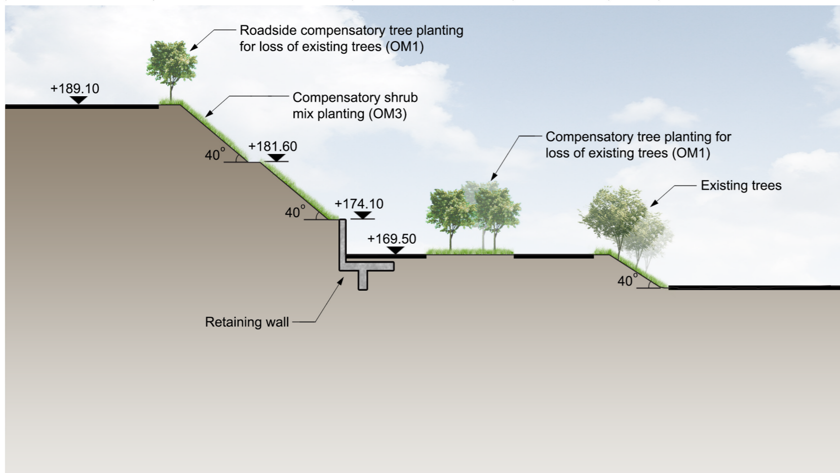
SECTION E - E
