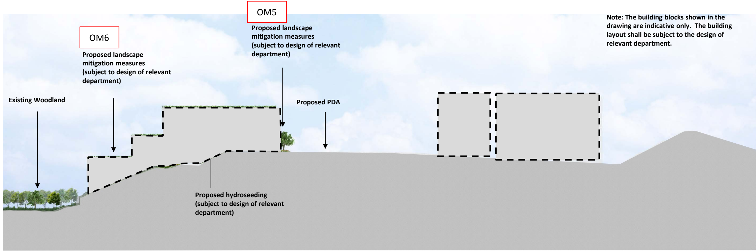
Section G-G N.T.S.
