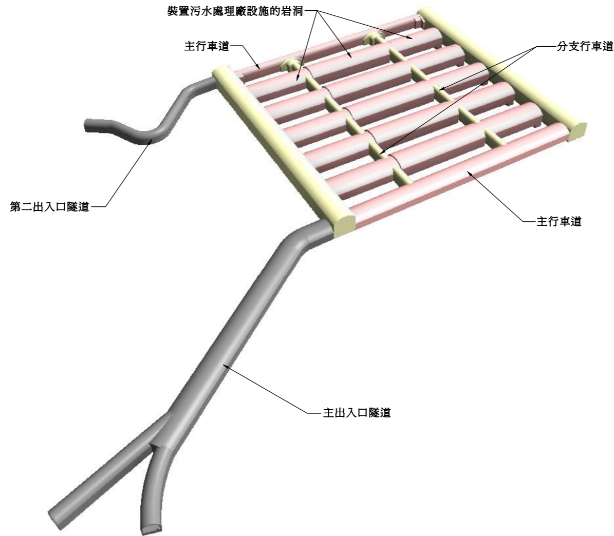
岩洞污水處理廠的3-D立體圖 (不按比例)
