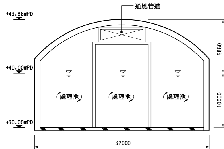
裝置污水處理廠設施的岩洞的典型剖面圖 比例 1 : 400
