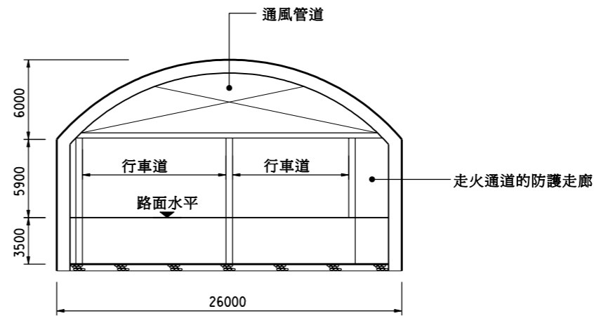
隧道的典型剖面圖 比例 1 : 400
